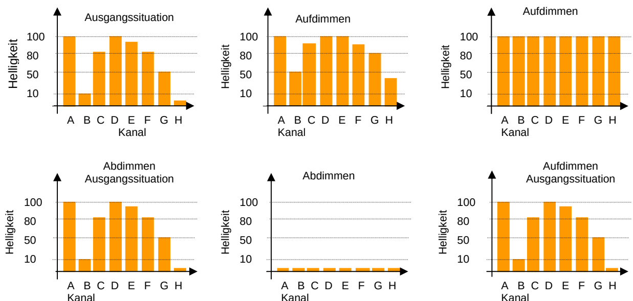
Abb. 8 Szenisches Dimmen mit Zentralbefehl
