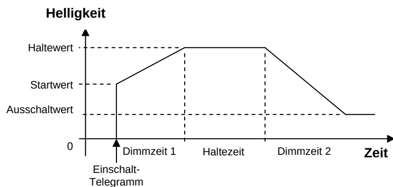
Abb. 7 Dynamik Betrieb - Zeitlicher Verlauf des Dimmbereichs
