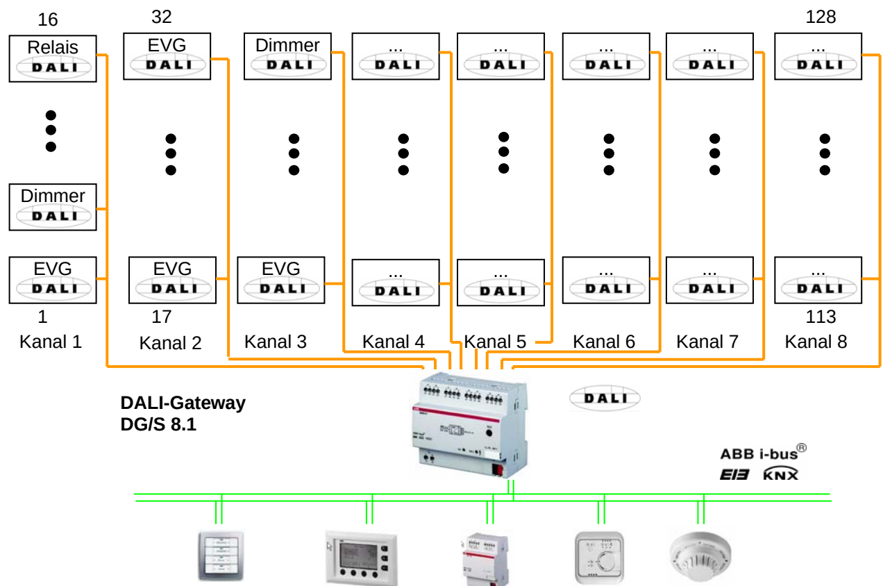
Abb. 3 DALI-Gateway DG/S 8.1 Prinzipschema
