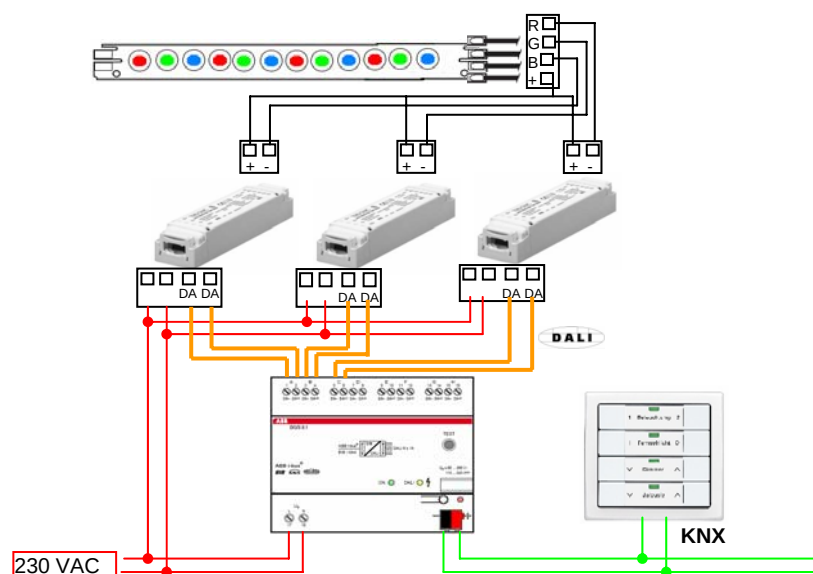
Abb. 28 Farbige LED Systembeispiel
