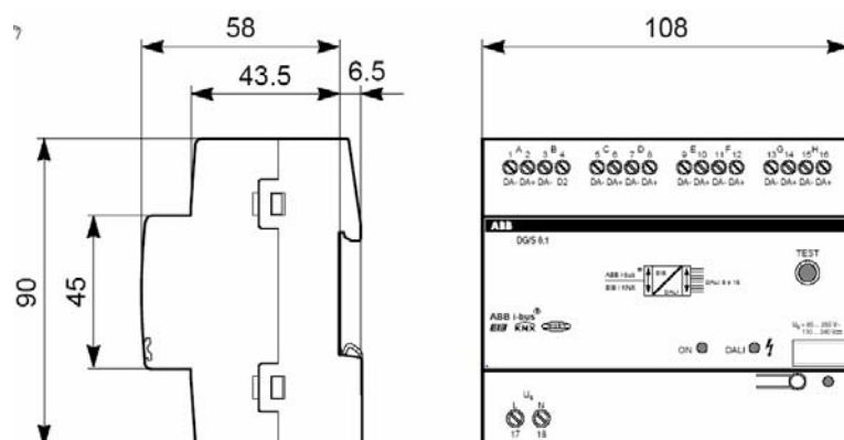
Abb. 5 DALI-Gateway DG/S 8.1 Maßbild
