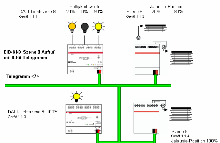
Abb. 27 8-Bit-Szene Beispiel: Aufruf Szene Nr. 8
