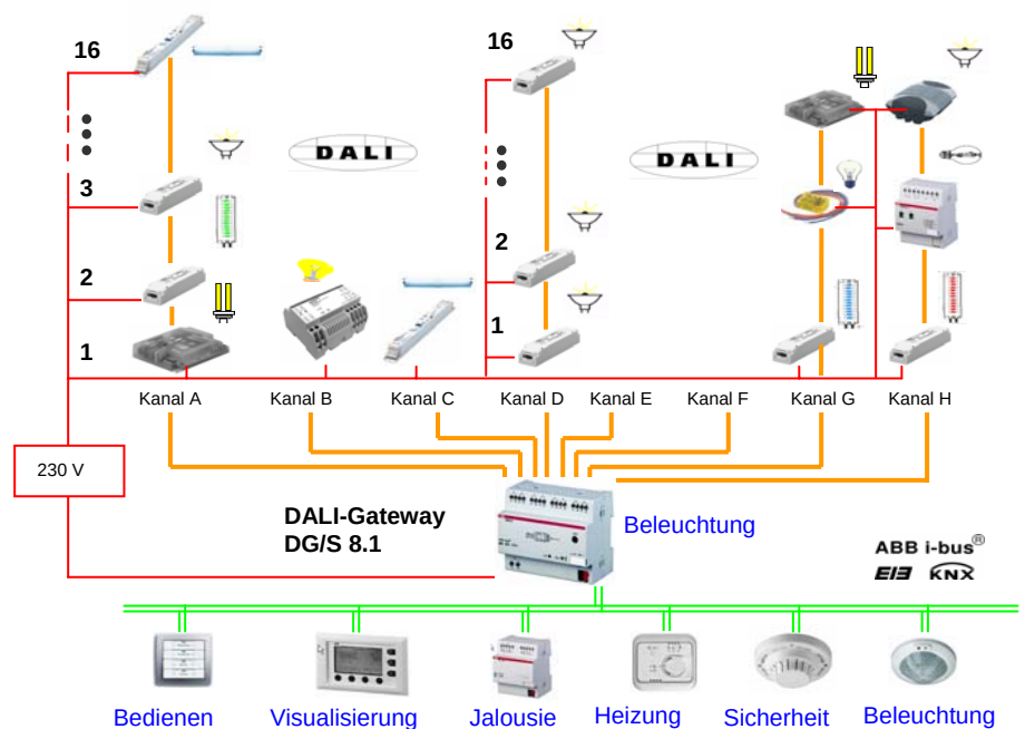
Abb. 6 DALI-Gateway DG/S 8.1 Anschlusschema
