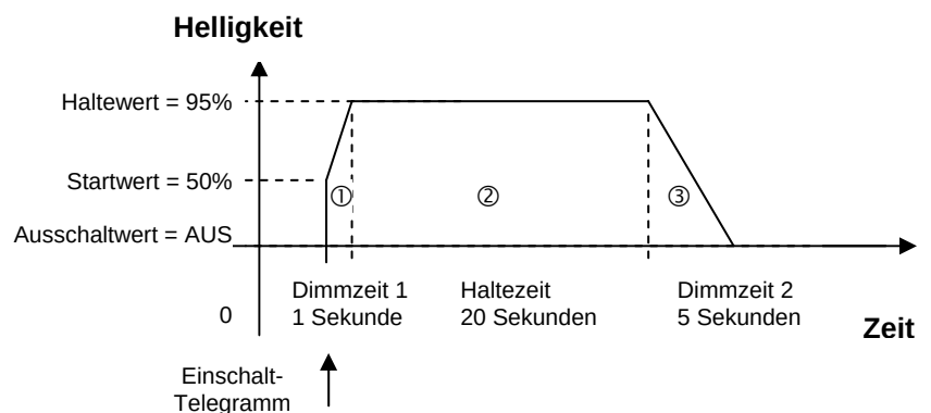
Abb. 30 Zeitlicher Verlauf Treppenlichtfunktion
