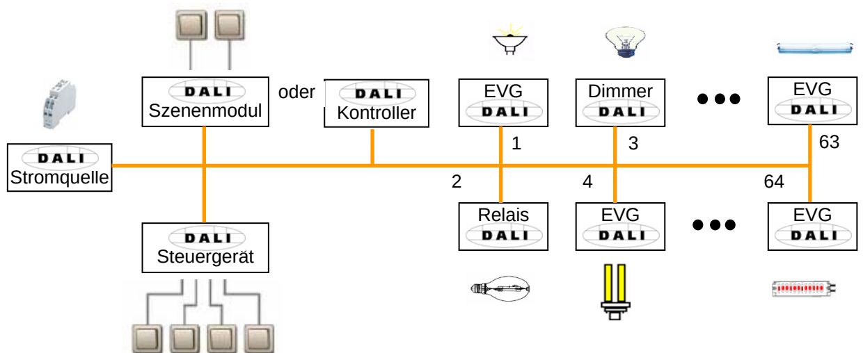
Abb. 2 DALI Prinzipschaltbild
