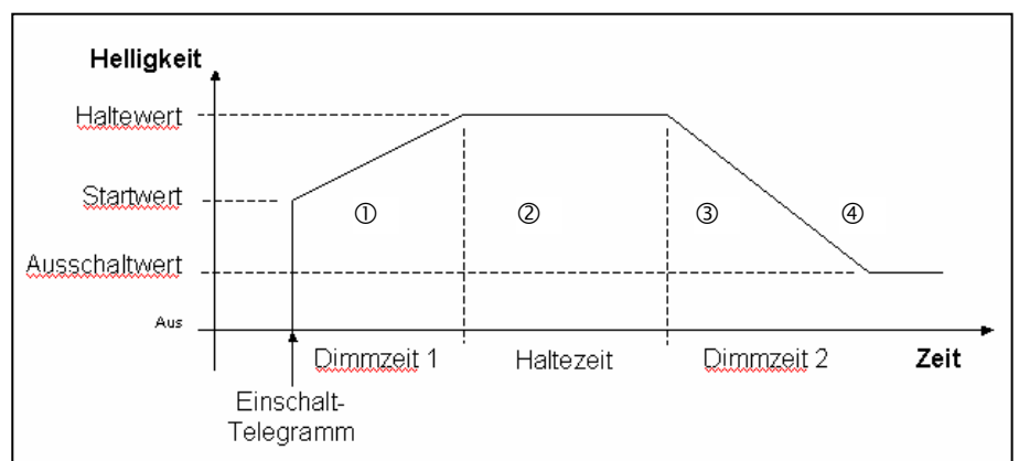
Abb. 22 Graphische Darstellung des Dynamik-Betrieb
