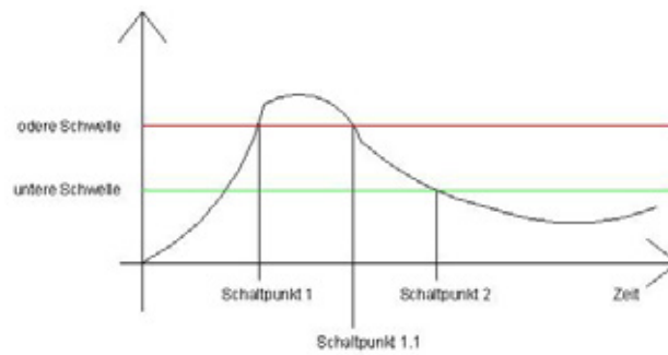
Abbildung 110: Diagramm Schwellwertschalter
