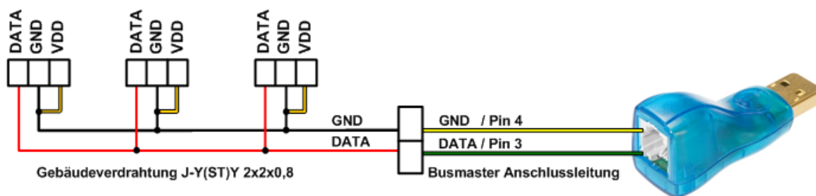
Abbildung 4: Installationsvariante 1-Wire-Sensoren mit „Parasitic Power“
