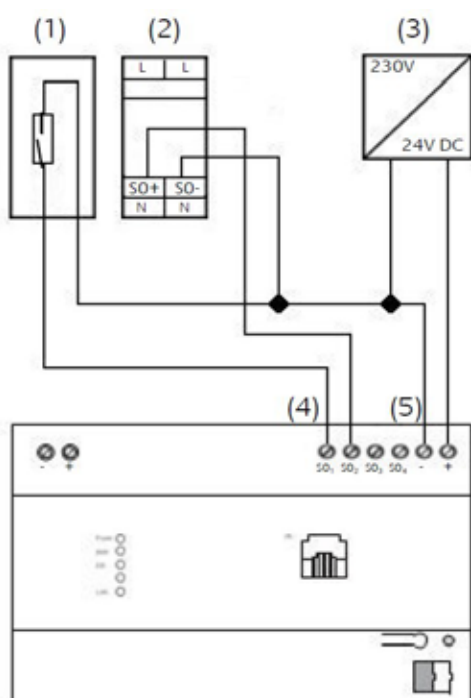
Abbildung 115: SO-Anschlussschema
