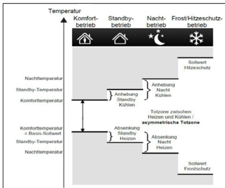
Abbildung 120 RTR - Job Funktionsschema
