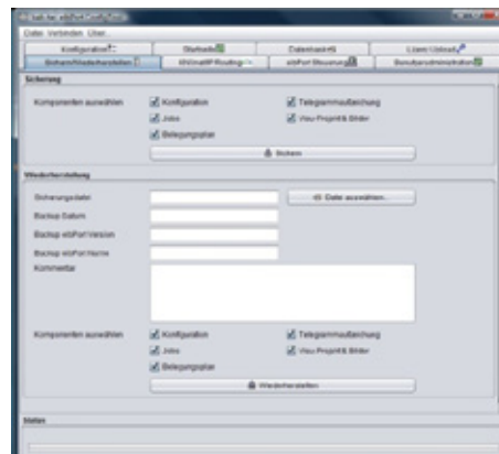
Abbildung 188: ConfigTool - Sichern/Wiederherstellen
