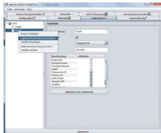
Abbildung 185: ConfigTool - Datenbankverbindung
