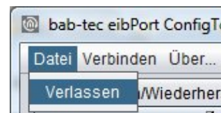
Abbildung 175: ConfigTool - Menüleiste
