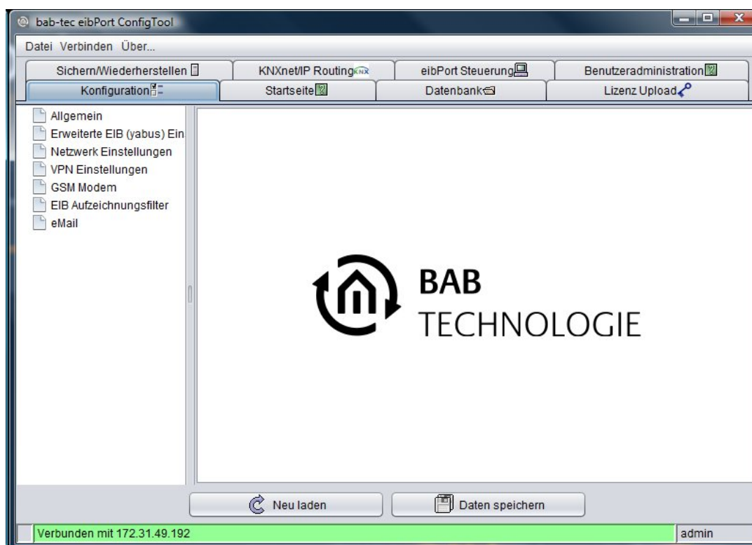
Abbildung 174: ConfigTool - Übersicht
