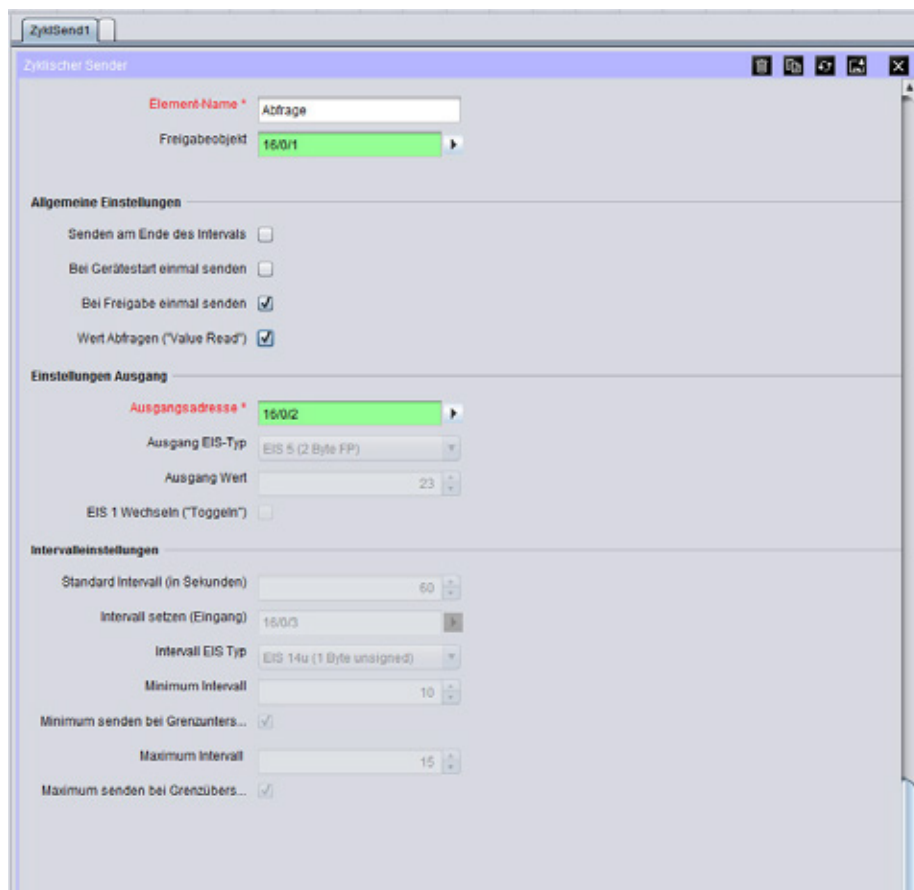
Abbildung 112: Zyklischer Sender - Anwendungsbeispiel
