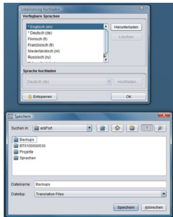
Abbildung 24: Editor - Lokalisierungsdialog
