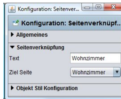
Abbildung 95: Seitenverknüpfung - Parameter
