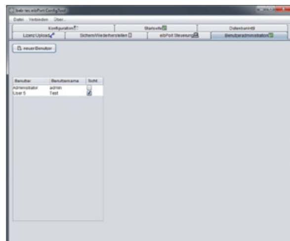
Abbildung 189: ConfigTool - Benutzeradministration
