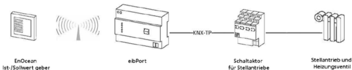
Abbildung 126: RTR Job -Anwendungsbeispiel
