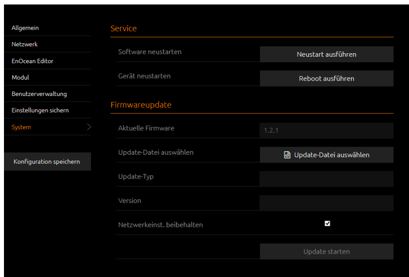
Abbildung 55: Konfiguration – System
