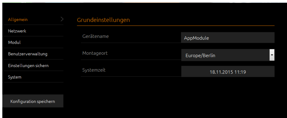
Abbildung 50: Allgemeine Konfigurationen
