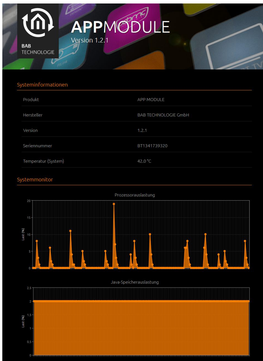
Abbildung 58: Information
