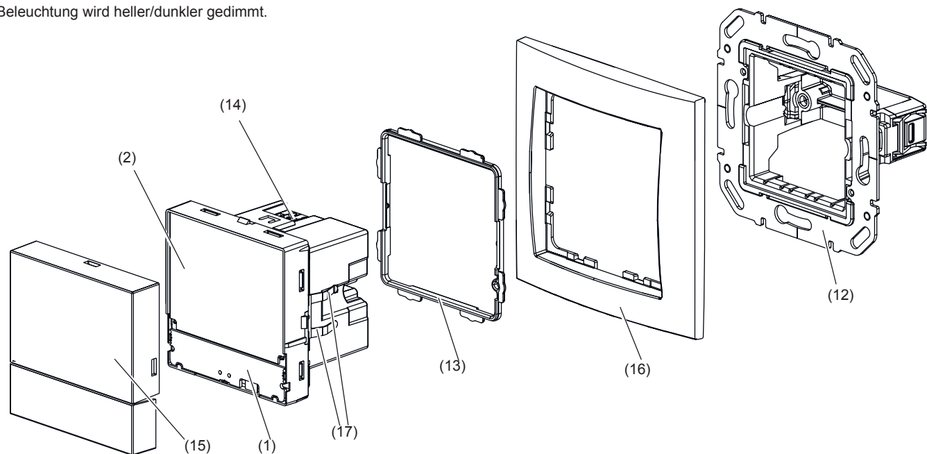
Bild 21: Gerät montieren
