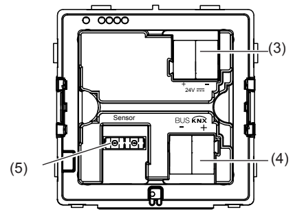
Bild 2: Rückansicht
