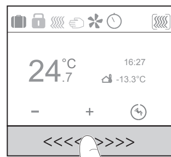
Bild 4: Slider-Funktion
