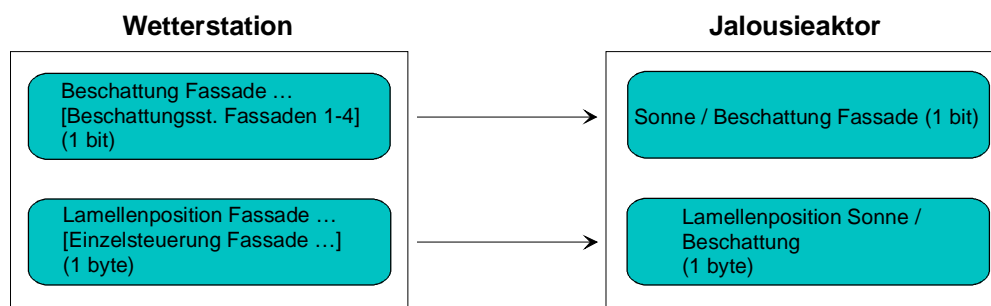
Bild 25: Projektierung der Kommunikationsobjekte für Anwendungsbeispiel III.
