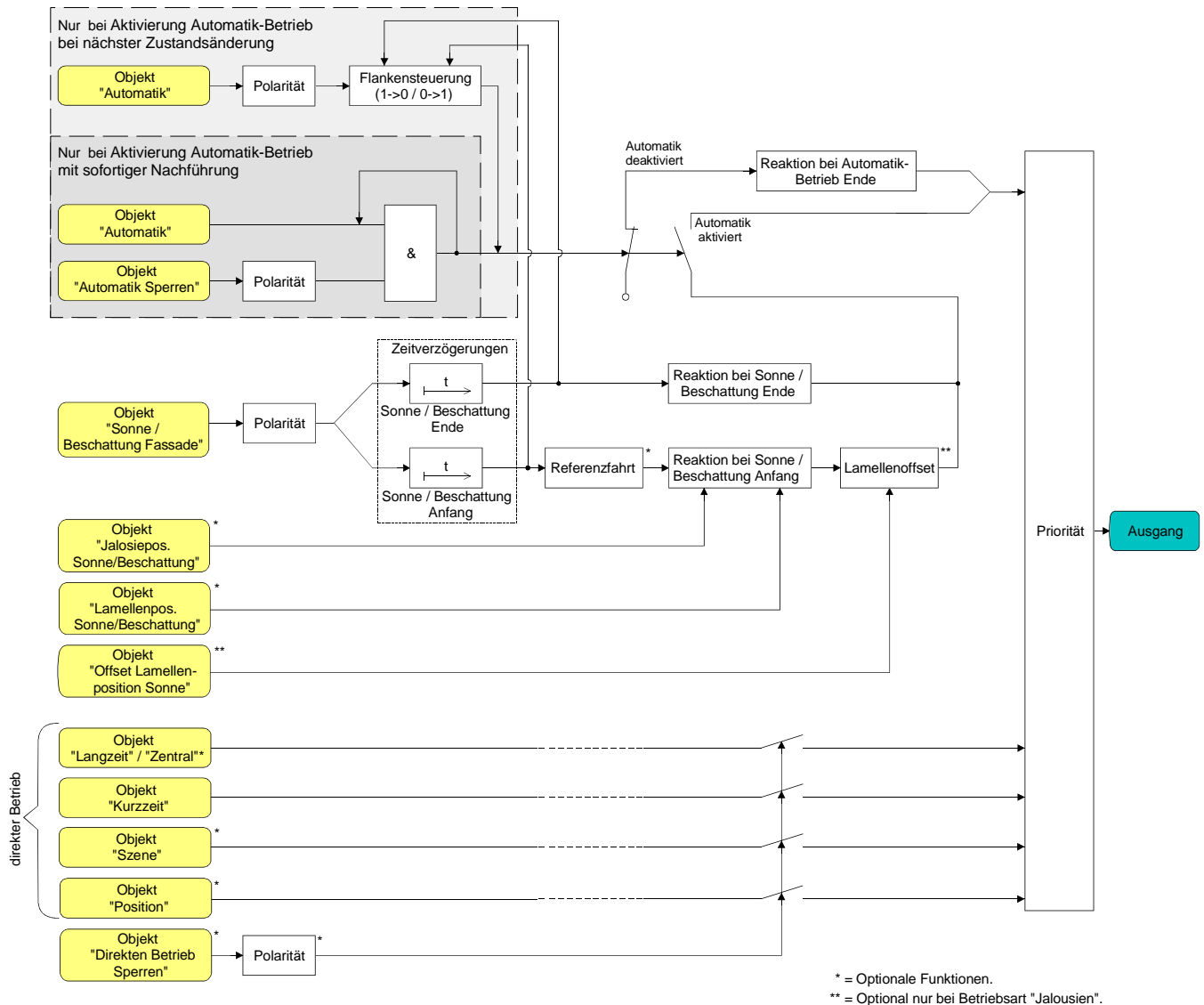
Bild 21: Funktionsschaltbild des erweiterten Sonnenschutzes
