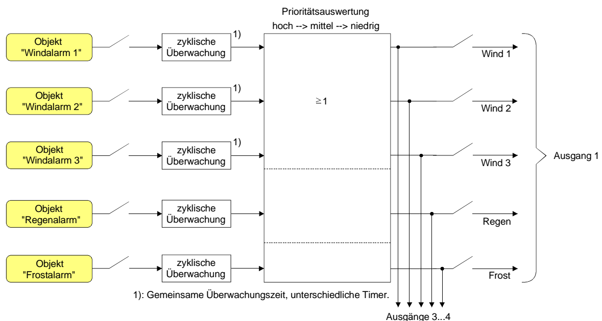
Bild 8: Funktionsschaltbild der Sicherheitsfunktionen
