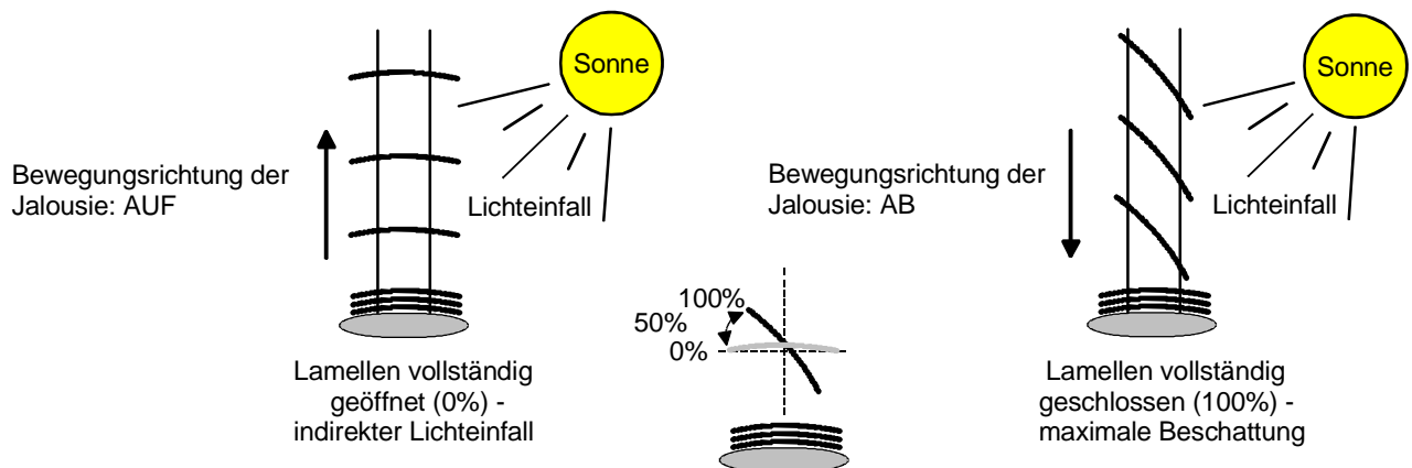
Bild 11: Typ 2 - Lamellenjalousien mit schräger und gerader Lamellenstellung
