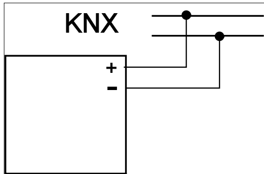
Anschluss an Twisted Pair
