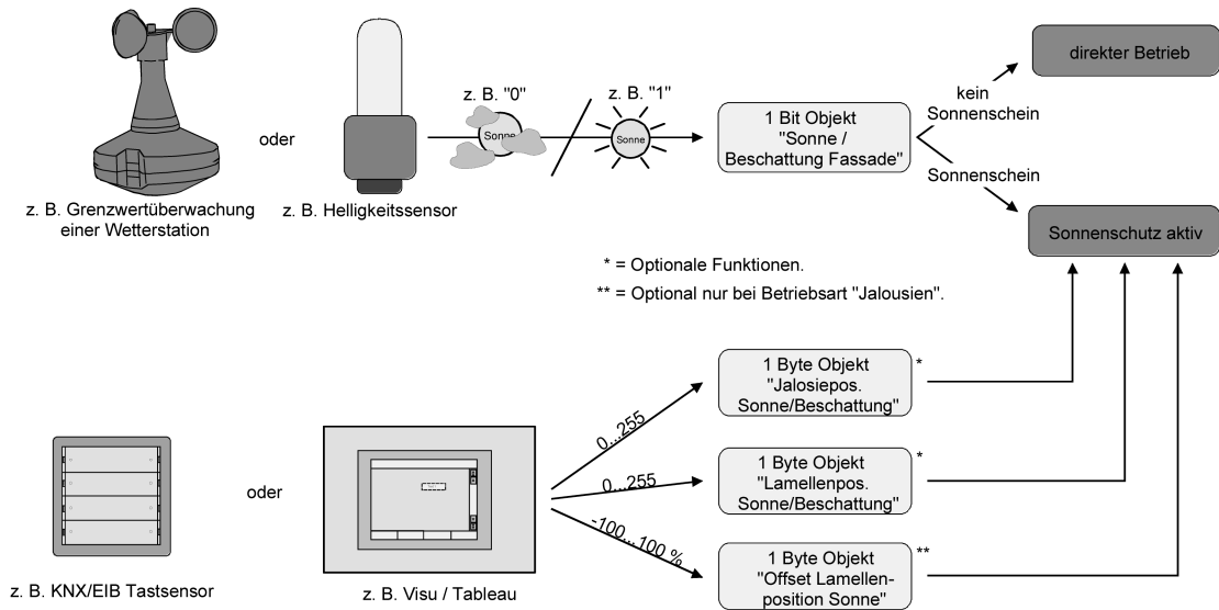
Bild 20: Prinzipialschaltbild des einfachen Sonnenschutzes
