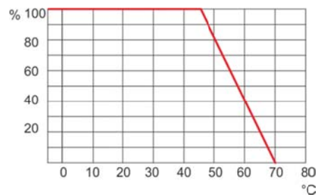
Abb. 2: Maximale Anschlussleistung in Abhängigkeit von der Umgebungstemperatur
