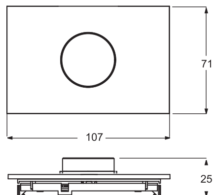
UP-Drehbedienelement 6341-xxx-101-500
