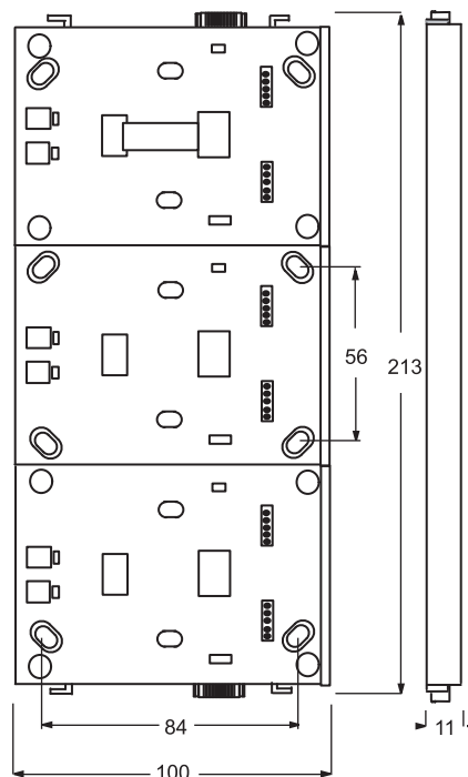
UP-Drehbedienelement 6341-xxx-101-500
