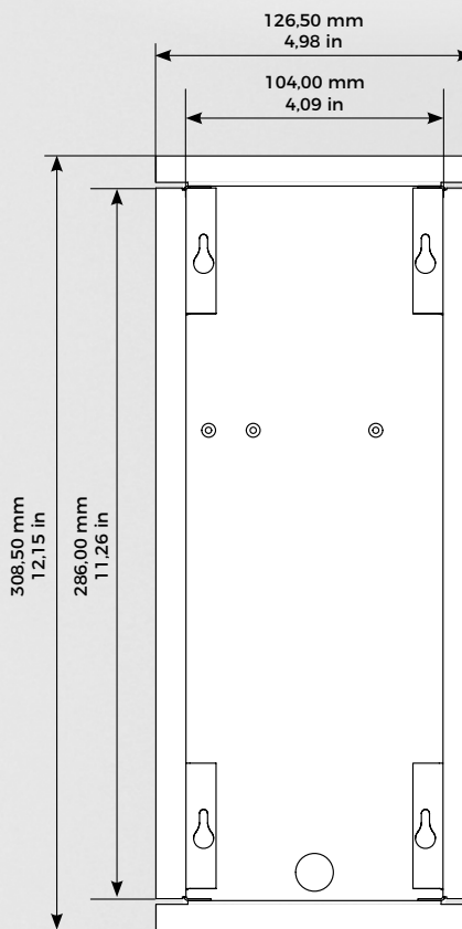
Unterputzgehäuse
