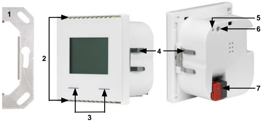
Abb. 2 1 Tragrahmen 2 Öffnungen für Luftzirkulation 3 Touch-Tasten 4 Rasten 5 Programmier-LED (versenkt) 6 Programmier-Taste (versenkt) zum Einlernen des Geräts
