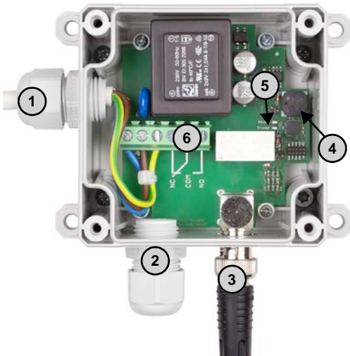
Abb. 4 Innenansicht
