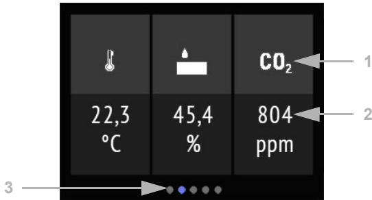
Abb. 12: Menü Sensorik, Beispiel Cala Touch KNX AQS/TH
