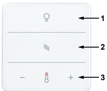
Abb. 2 Vorderseite 1 Bereich „Licht“ mit 3 Touch-Flächen 2 Bereich „Sonnenschutz/Antrieb“ mit 3 Touch-Flächen 3 Bereich „Temperatur“ mit 3 Touch-Flächen
