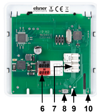
Abb. 4 Rückansicht ohne Halterung 6 KNX-Busklemme +/- für Anschluss bei Montage über einer Dose 7 Federkraftklemmen KNX-Bus für flächenbündige Montage direkt auf der Wand 8 Programmier-Taste (versenkt) zum Einlernen 9 Programmier-LED 10 Temperatursensor PRG-Taste ist bei montiertem Gerät erreichbar von unten/außen (siehe Kapitel Gerät adressieren).
