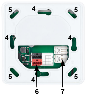
Abb. 3 Rückansicht mit Halterung 4/5 Schraublöcher für verschiedene Dosen. Die Befestigung mit 2 Schrauben ist ausreichend. Verwenden Sie bei Wandmontage ein für den Untergrund geeignetes Befestigungsmaterial! 6 KNX-Busklemme +/- für Anschluss bei Montage über einer Dose 7 Federkraftklemmen KNX-Bus für flächenbündige Montage direkt auf der Wand
