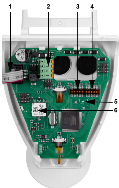
Abb. 11: Übersicht Platine
