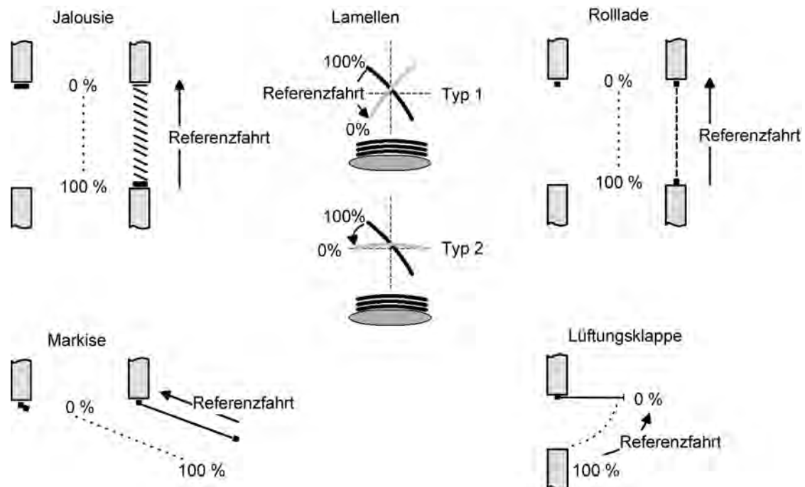
Bild 20: Referenzfahrt
