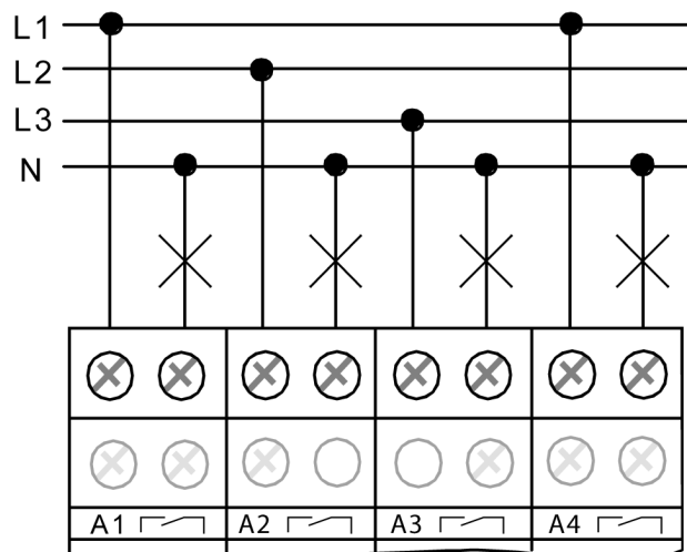
Bild 6: Elektrischer Anschluss für Lasten im Schaltbetrieb
