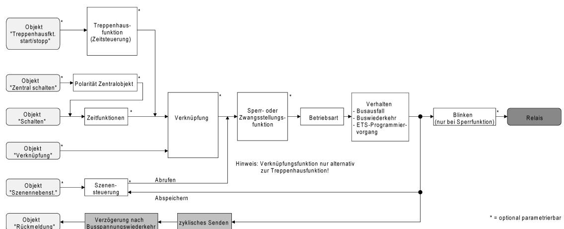
Bild 17: Funktionsschaltbild der Rückmeldung
