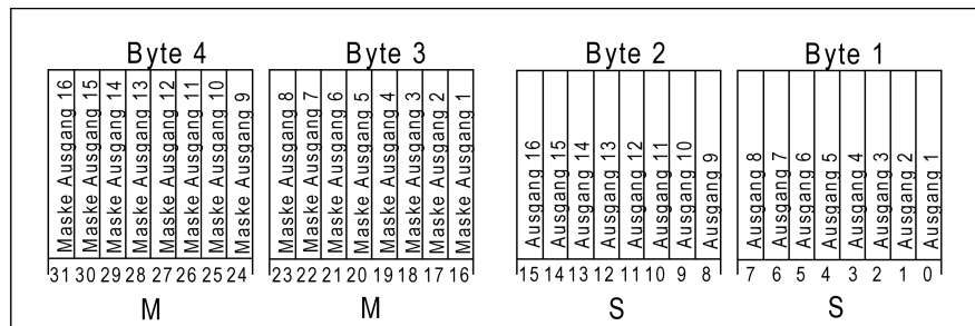
Bild 14: Struktur des Objektes der Sammelrückmeldung
