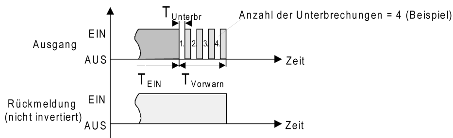
Bild 22: Die Vorwarnfunktion der Treppenhausfunktion (Beispiel)
