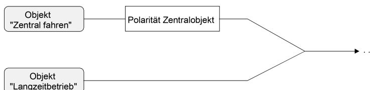
Bild 13: Funktionsschaltbild "Zentral fahren"
