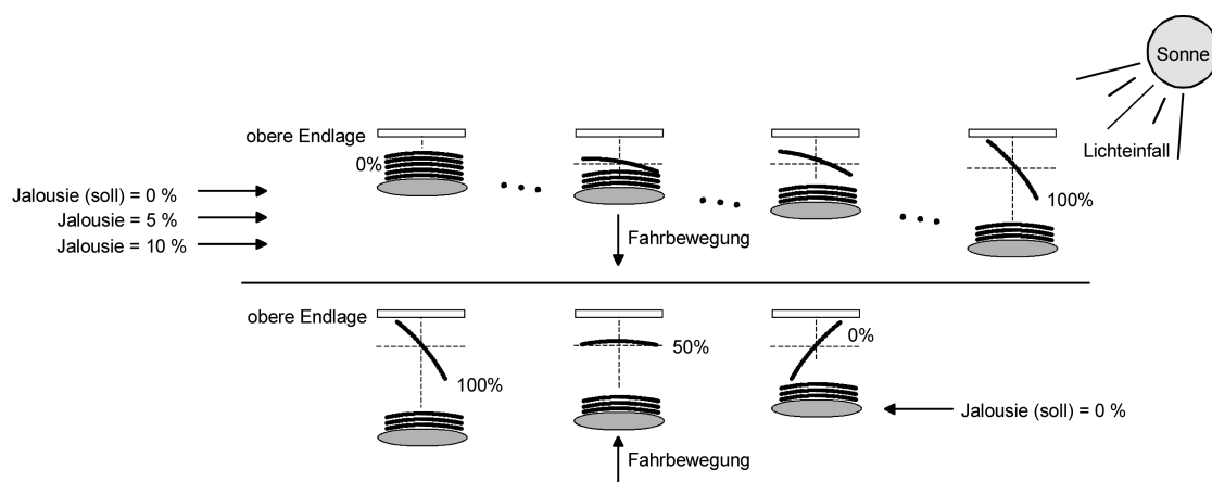
Bild 33: Beispiel für Lamellenpositionierung bei Jalousieposition in der oberen Endlage (Beispielhaft für Lamellentyp 1.)
