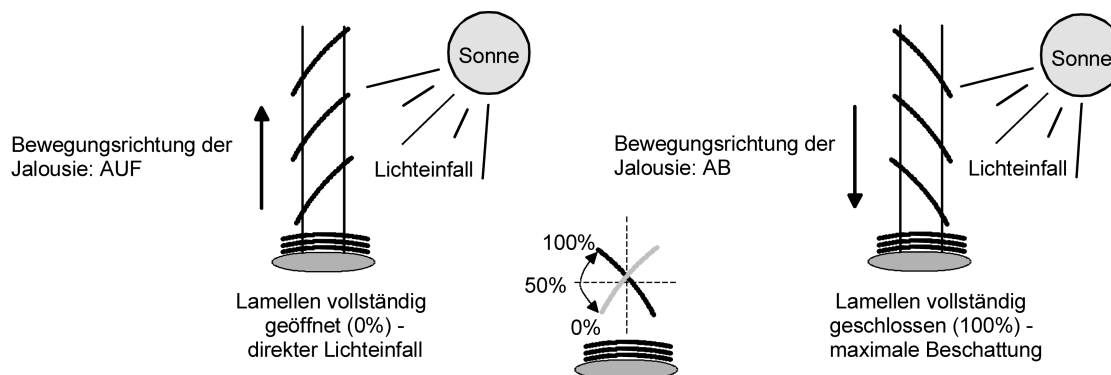
Bild 29: Typ 1 - Lamellenjalousien mit schräger Lamellenstellung in beide Fahrtrichtungen
