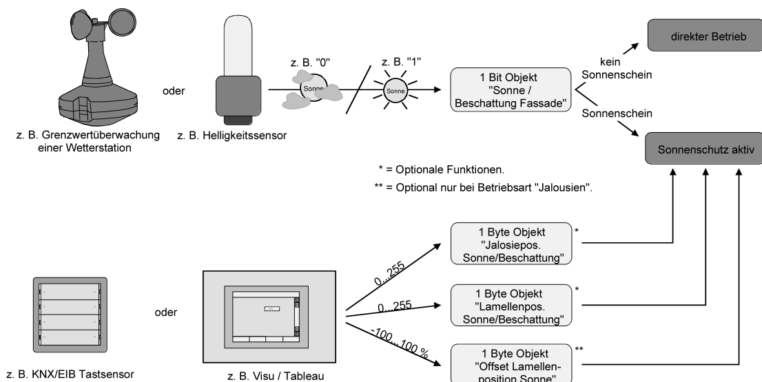
Bild 37: Prinzipschaltbild des Sonnenschutzes
