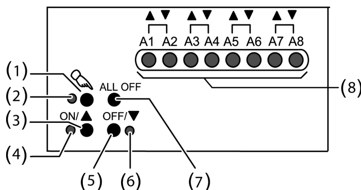
Bild 10: Bedien- und Anzeigeelemente der Handbedienung beim Schalt-/Jalousieaktor 4/8fach
