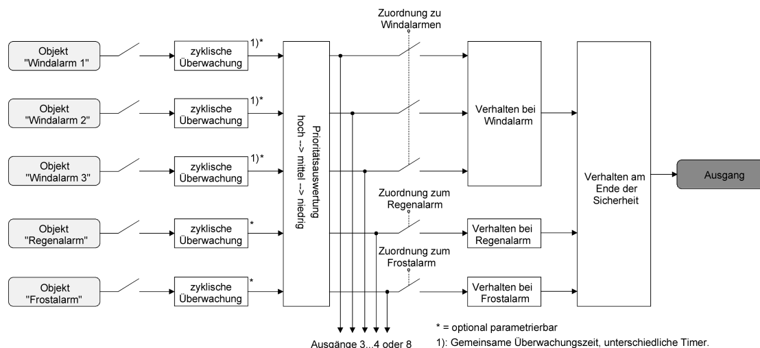
Bild 35: Funktionsschaltbild der kanalorientierten Sicherheitsfunktionen
