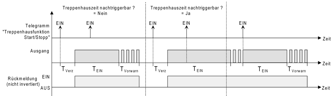
Bild 20: Einschaltverhalten der Treppenhausfunktion
