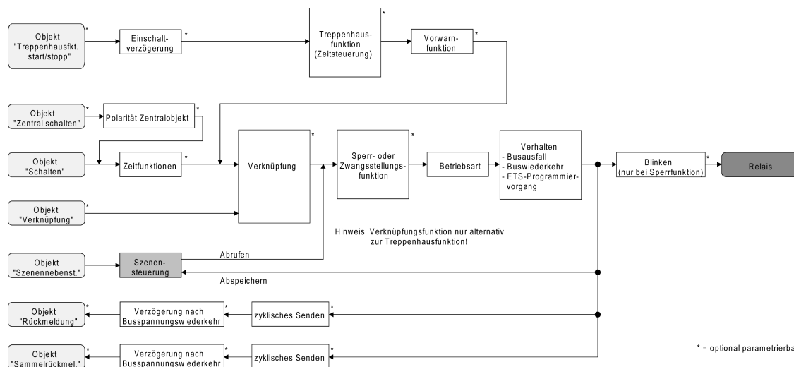
Bild 23: Funktionsschaltbild der Szenenfunktion
