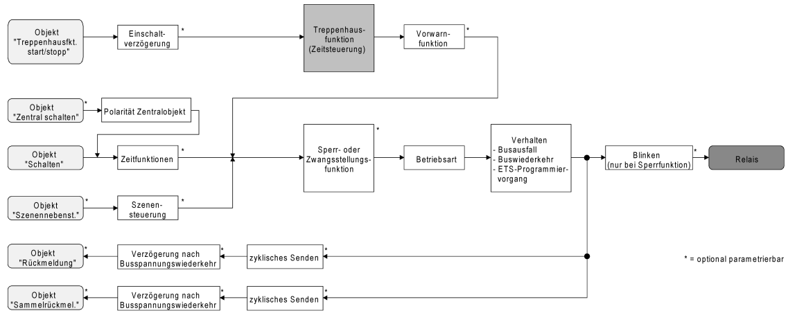
Bild 19: Funktionsschaltbild der Treppenhausfunktion
