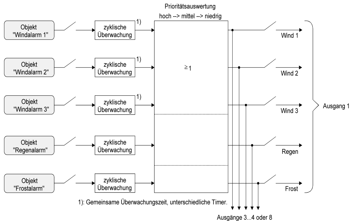
Bild 15: Funktionsschaltbild der Sicherheitsfunktionen
