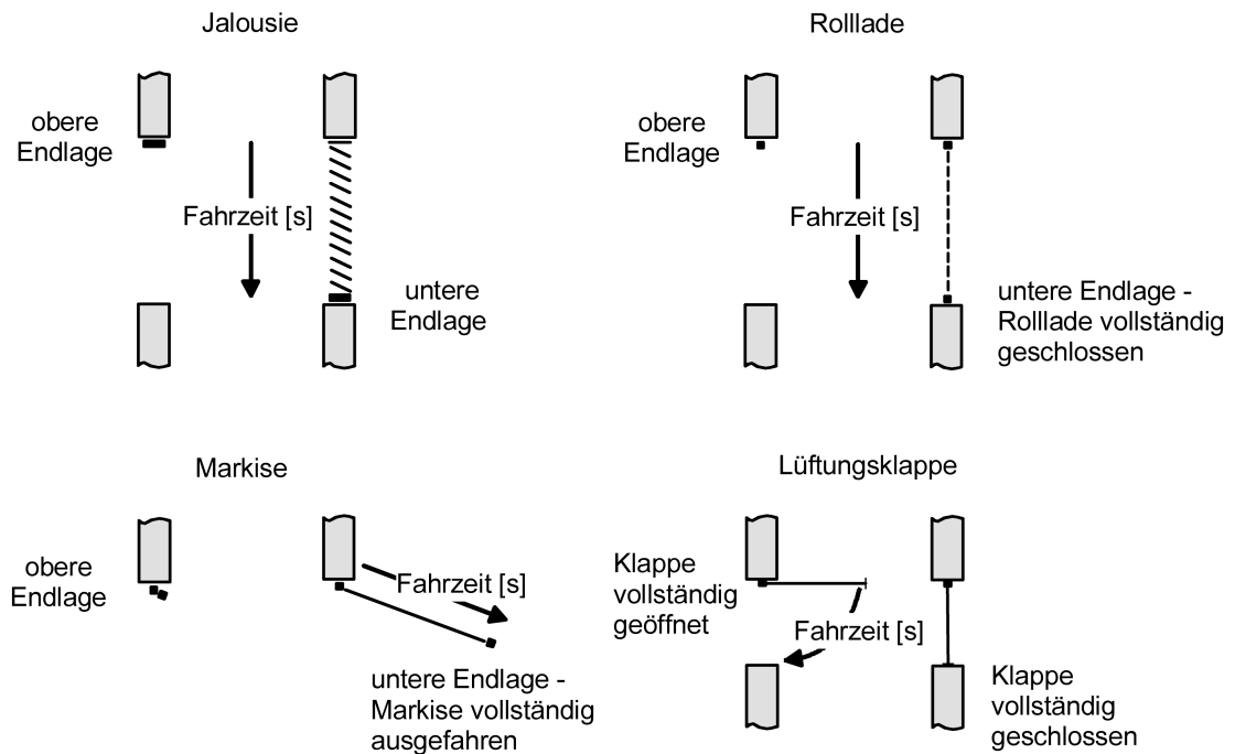
Bild 28: Ermittlung der Fahrzeit in Abhängigkeit der Antriebsart
