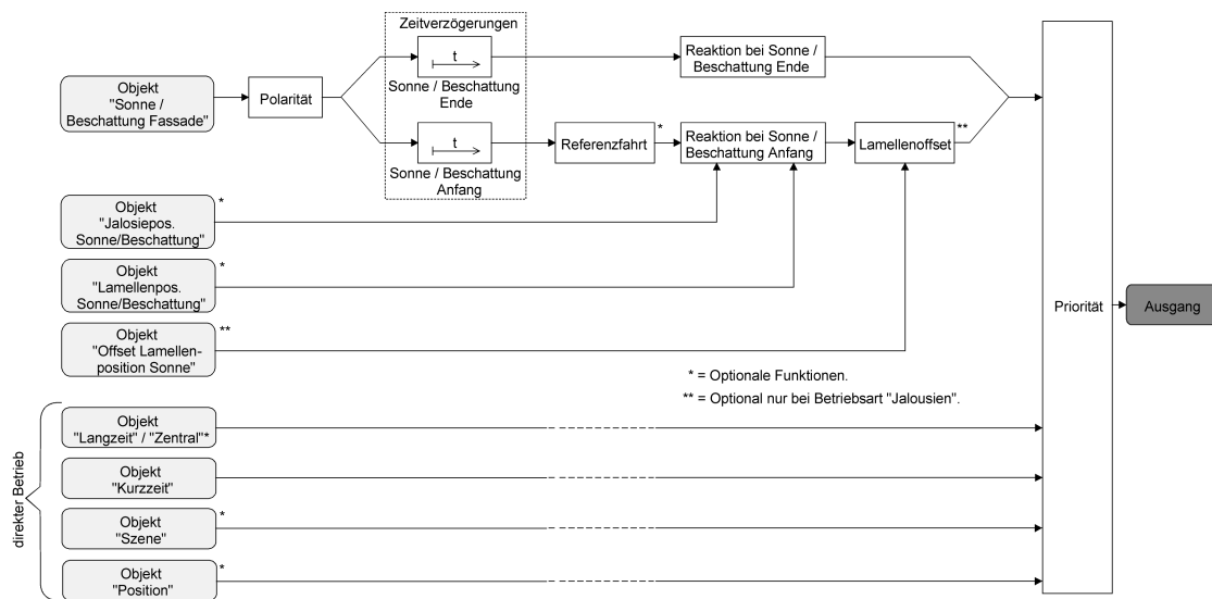
Bild 38: Funktionsschaltbild des Sonnenschutzes
