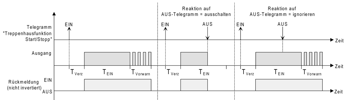
Bild 21: Ausschaltverhalten der Treppenhausfunktion
