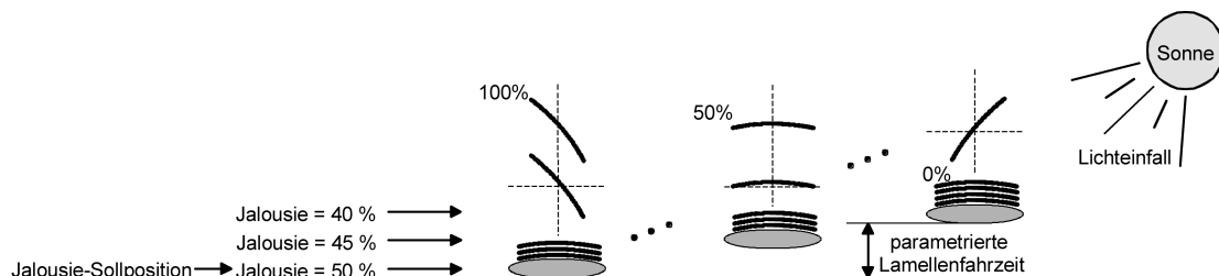
Bild 32: Beispiel für Lamellenpositionierung mit Auswirkung auf die Jalousieposition (Beispielhaft für Lamellentyp 1. Typ 2 sinngemäß gleich.)
