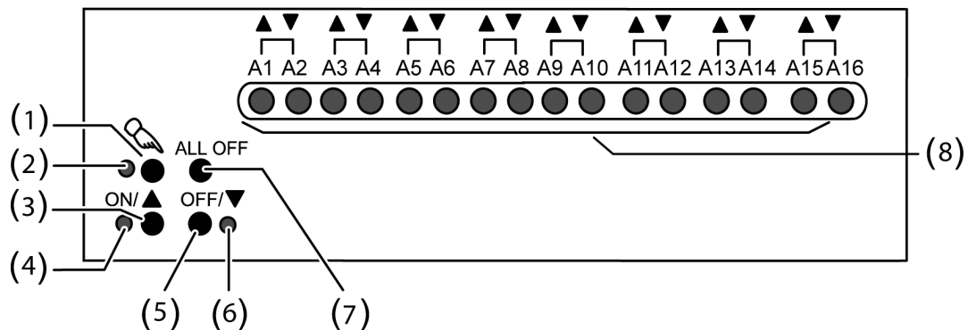
Bild 11: Bedien- und Anzeigeelemente der Handbedienung beim Schalt-/Jalousieaktor 8/16fach
