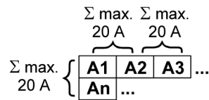
Bild 7: Summenstrombelastbarkeit benachbarter Ausgänge
