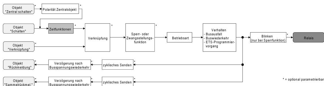
Bild 18: Funktionsschaltbild der Zeitverzögerungen
