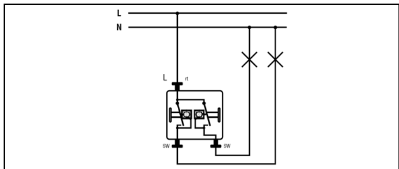
Anschlussbeispiel 535 U5
