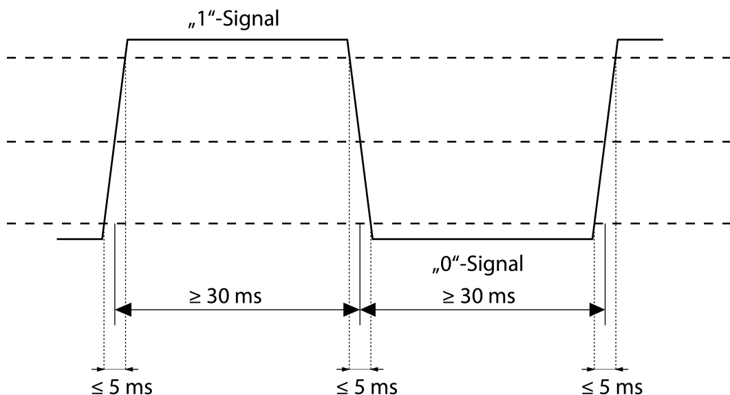
Bild 9: Signalverlauf S0-Impuls
