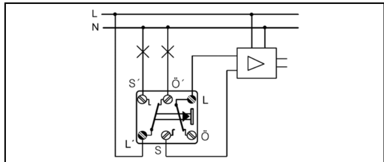
Anschlussbeispiel 533-2 U
