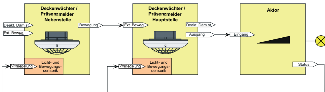
Bild 31: Applikationsbeispiel Haupt- und Nebenstelle ohne Dämmerungsstufenauswertung
