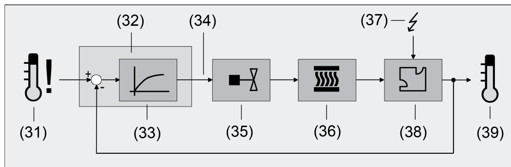
Bild 43: Regelstrecke einer Einzelraum-Temperaturregelung
