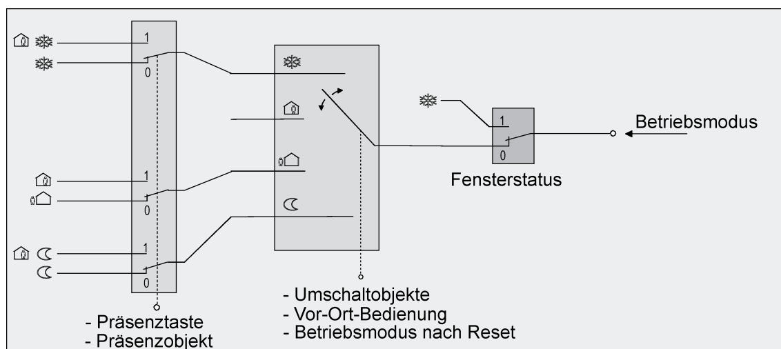
Bild 52: Betriebsmodusumschaltung durch 4 x 1 Bit Objekte mit Präsenztaste
