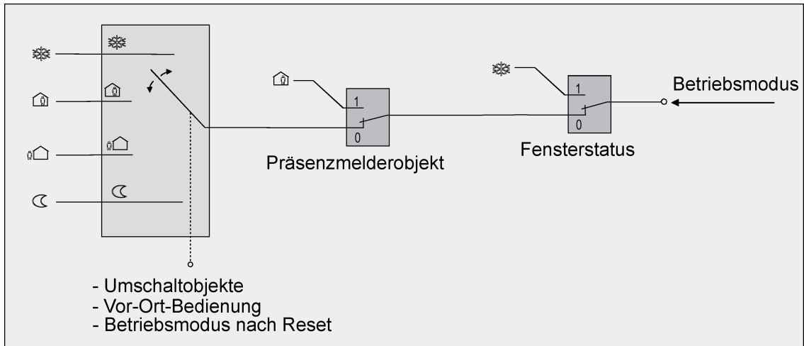
Bild 53: Betriebsmodusumschaltung durch 4 x 1 Bit Objekte mit Präsenzmelder
