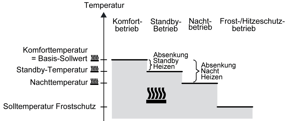
Bild 56: Solltemperaturen in der Betriebsart "Heizen"
