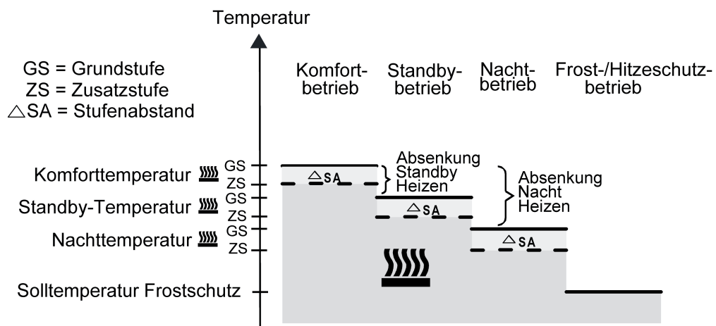
Bild 57: Solltemperaturen in der Betriebsart "Grund- und Zusatzheizen"
