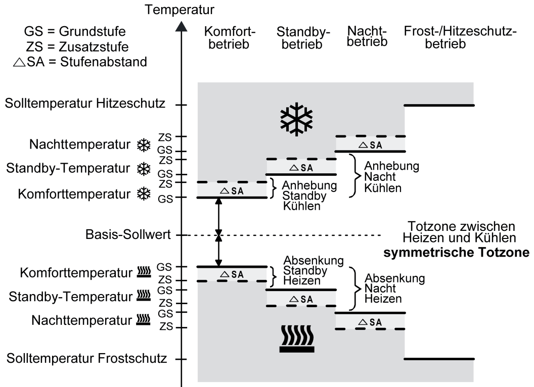
Bild 62: Solltemperaturen in der Betriebsart "Grund- und Zusatzheizen und -kühlen" mit symmetrischer Totzone
