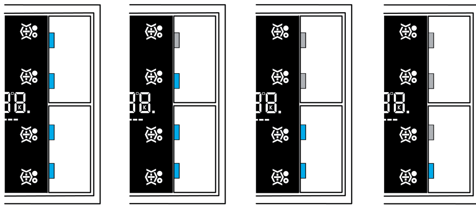
Bild 73: Standard Anzeigefunktion: negative Sollwertverschiebung "4 Schritte"
