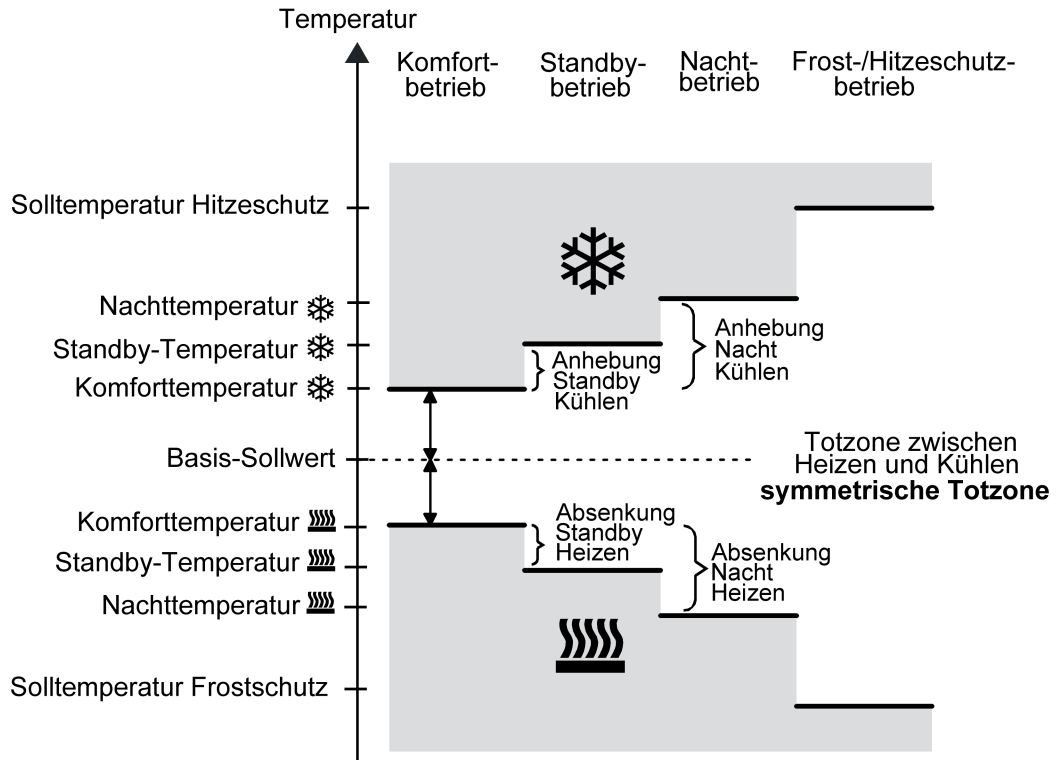
Bild 60: Solltemperaturen in der Betriebsart "Heizen und Kühlen" mit symmetrischer Totzone
