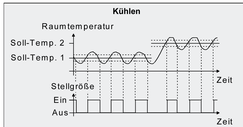
Bild 47: 2-Punkt-Regelung für Einzelbetriebsart "Kühlen"
