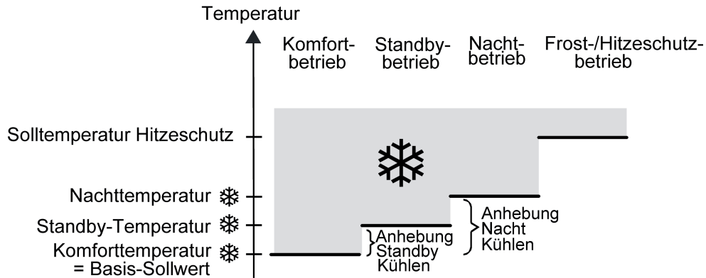
Bild 58: Solltemperaturen in der Betriebsart "Kühlen"
