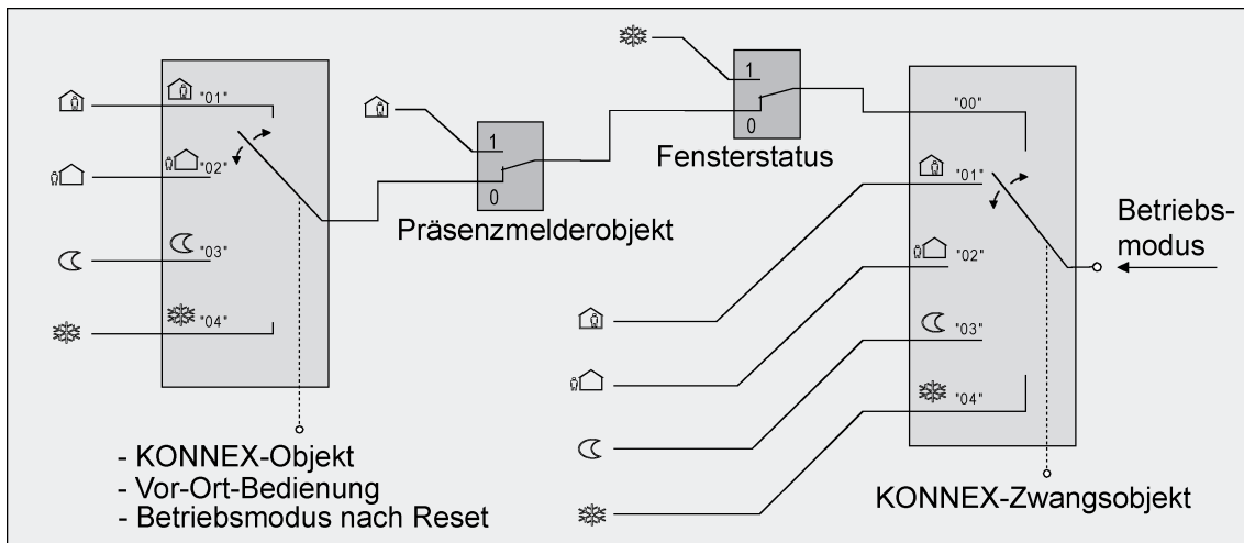
Bild 55: Betriebsmodusumschaltung durch KÖNNEX Objekt mit Präsenzmelder
