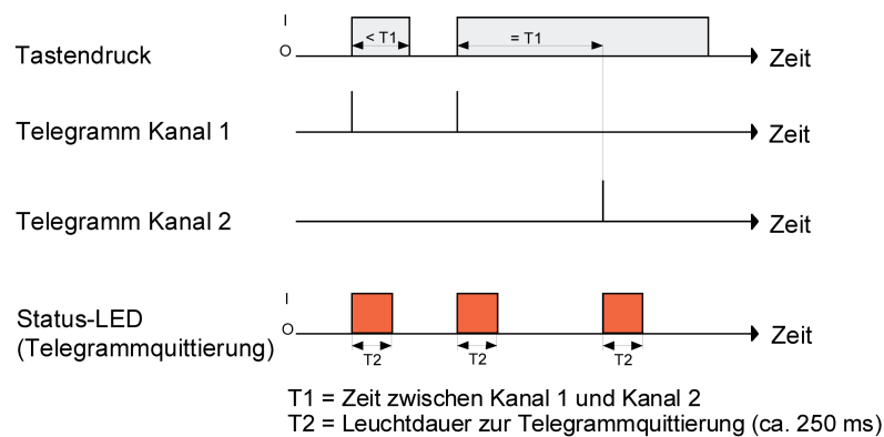
Bild 72: Beispiel zum Bedienkonzept "Kanal 1 oder Kanal 2"
