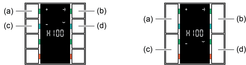
Bild 12: Tastenfunktionen innerhalb der Menüebene (links: Gerätevariante 4fach, rechts: Gerätevariante 2fach)
