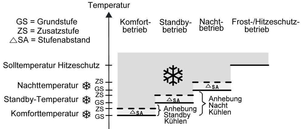
Bild 59: Solltemperaturen in der Betriebsart "Grund- und Zusatzkühlen"
