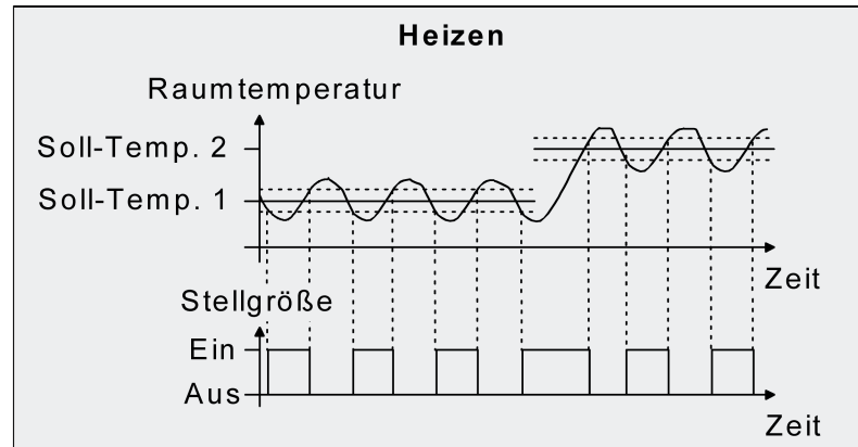
Bild 46: 2-Punkt-Regelung für Einzelbetriebsart "Heizen"
