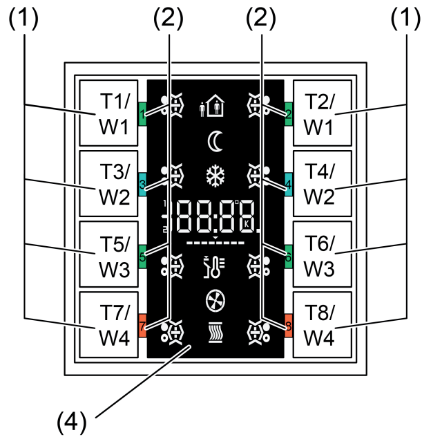
Bild 4: Frontansicht Kompakt-Raumcontroller-Modul 4fach (Display: Schalterprogramm LS990 & CD500)
