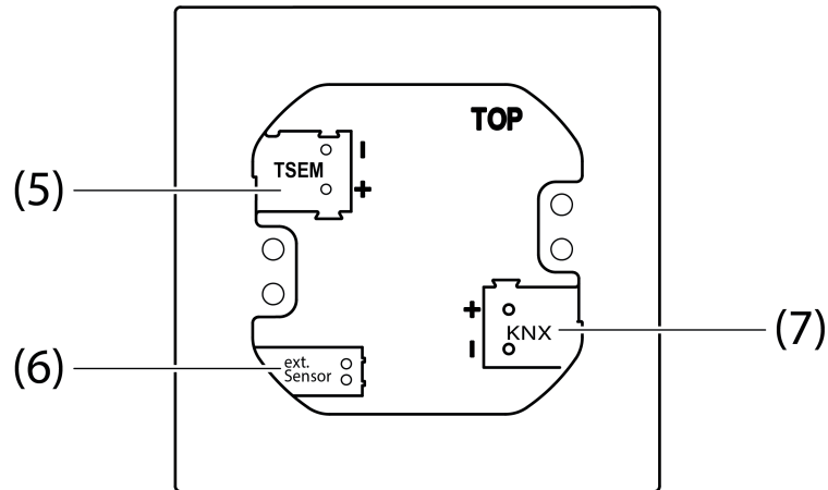
Bild 5: Rückseite Kompakt-Raumcontroller-Modul 2fach/4fach
