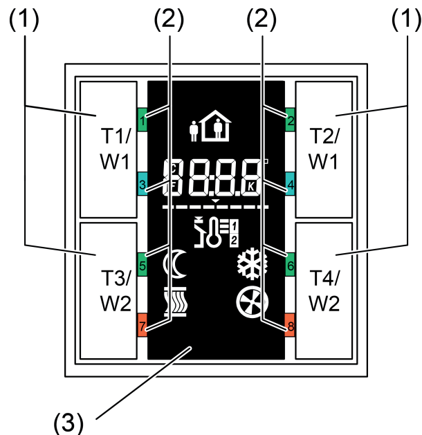
Bild 1: Frontansicht Kompakt-Raumcontroller-Modul 2fach (Display: Schalterprogramm A500)
