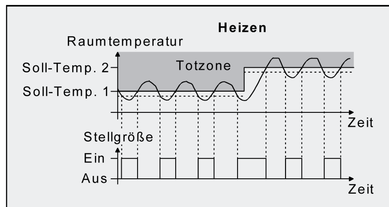
Bild 48: 2-Punkt-Regelung für Mischbetriebsart "Heizen und Kühlen" bei aktivem Heizbetrieb
