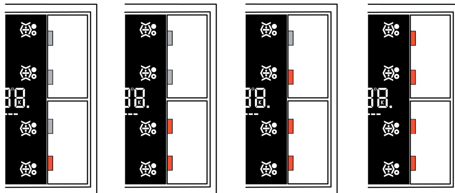
Bild 74: Standard Anzeigefunktion: positive Sollwertverschiebung "4 Schritte"
