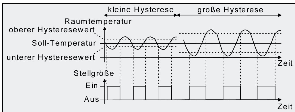
Bild 51: Auswirkungen der Hysterese auf das Schaltverhalten der Stellgröße einer 2-Punkt-Regelung
