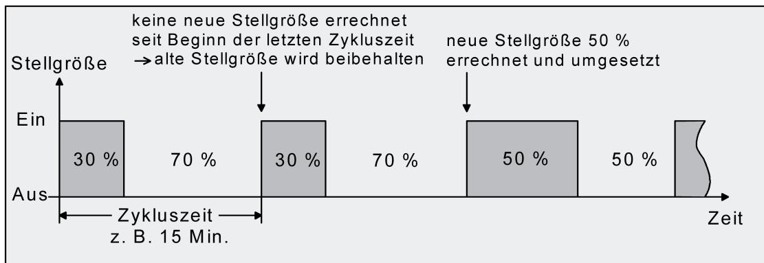
Bild 45: Schaltende PI-Regelung
