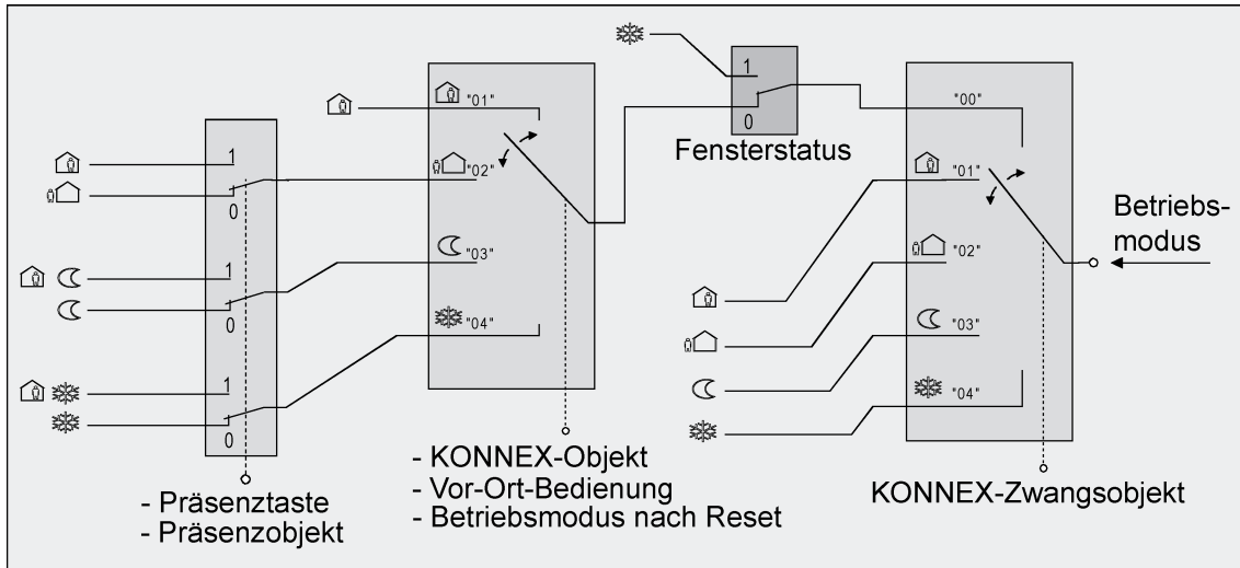
Bild 54: Betriebsmodusumschaltung durch KÖNNEX Objekt mit Präsenztaste
