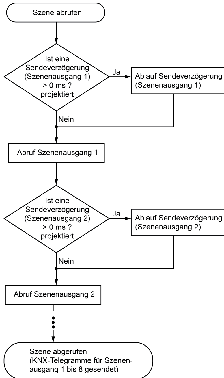
Bild 77: Flussdiagramm zur Sendeverzögerung einen Szenenausgangs
