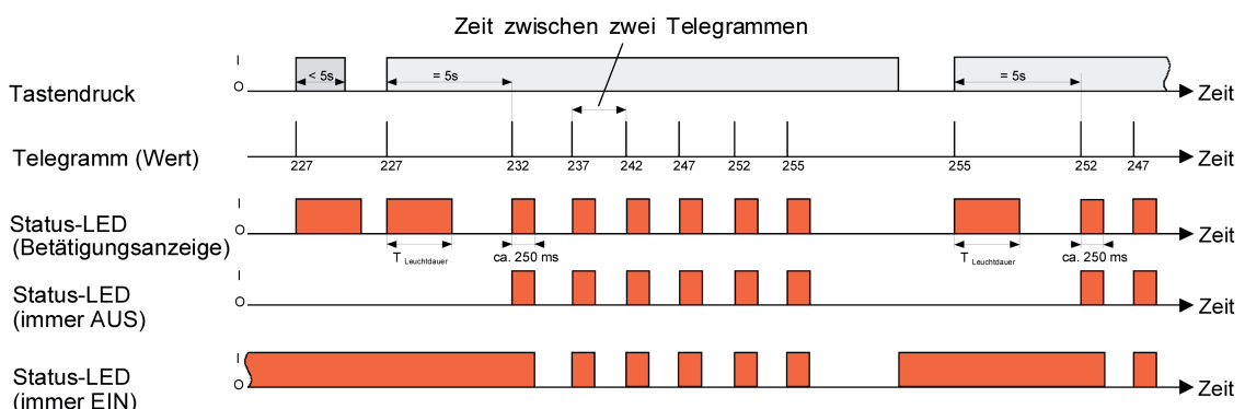
Bild 69: Beispiel zur Wertverstellung ohne Wertbereichs-Überlauf
