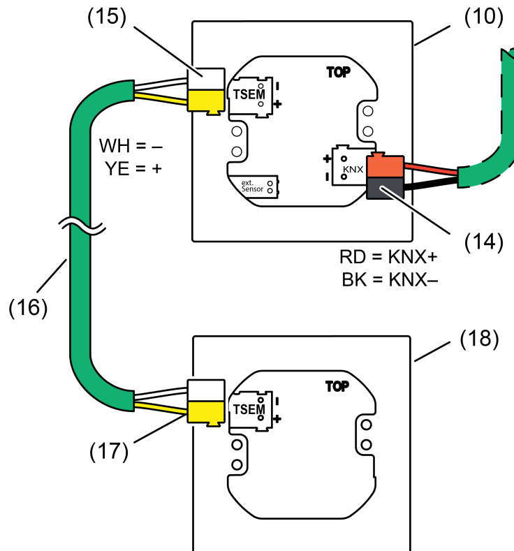
Bild 7: Anschluss des Tastensensor-Erweiterungsmoduls alternativ: Raumcontroller-Erweiterungsmodul (Ansicht von hinten)
