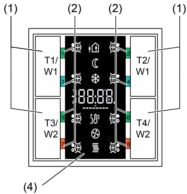
Bild 2: Frontansicht Kompakt-Raumcontroller-Modul 2fach (Display: Schalterprogramm LS990 & CD500)
