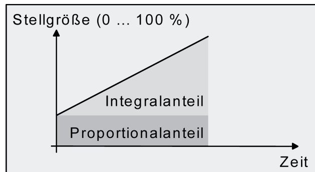
Bild 44: Stetige PI-Regelung
