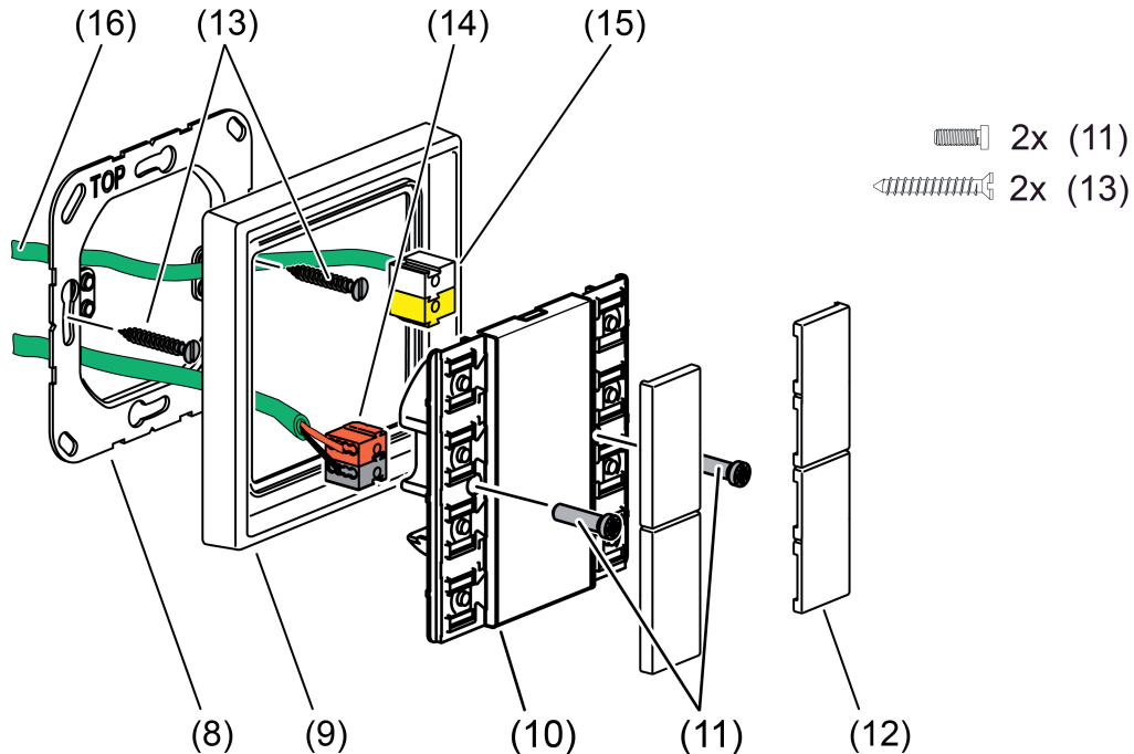
Bild 8: Montage des Kompakt-Raumcontroller-Moduls mit Anschluss eines Erweiterungsmoduls
