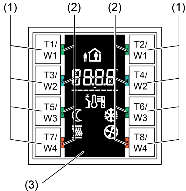
Bild 3: Frontansicht Kompakt-Raumcontroller-Modul 4fach (Display: Schalterprogramm A500)
