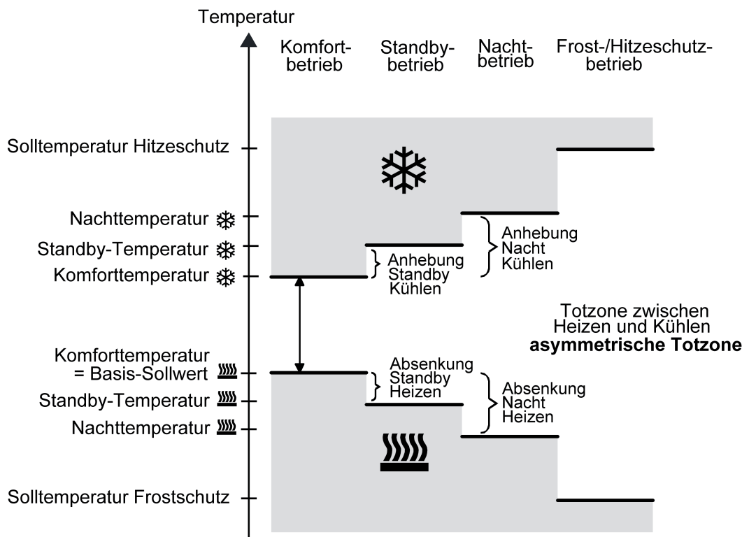
Bild 61: Solltemperaturen in der Betriebsart "Heizen und Kühlen" mit asymmetrischer Totzone
