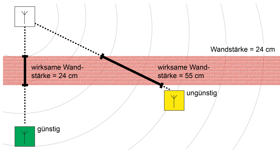
Bild 6: Dämpfung durch wirksame Wand- oder Deckenstärke
