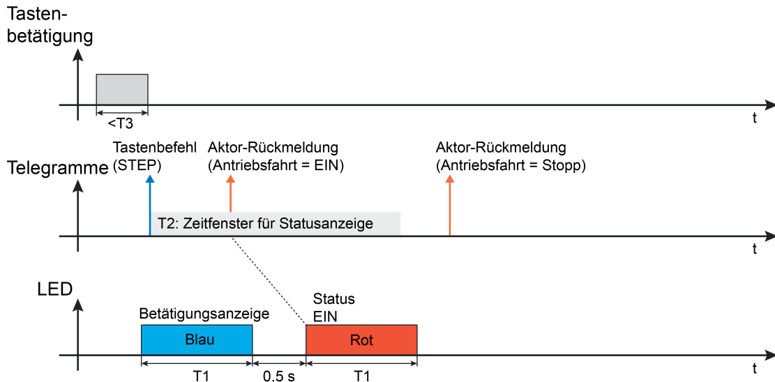
Bild 17: Beispiel einer Statusanzeige der Bedienfunktion "Jalousie" bei einem kurzen Tastendruck
