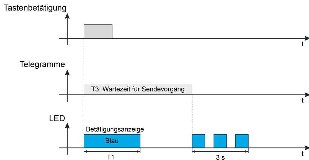
Bild 11: LED-Anzeige bei einem Übertragungsfehler
