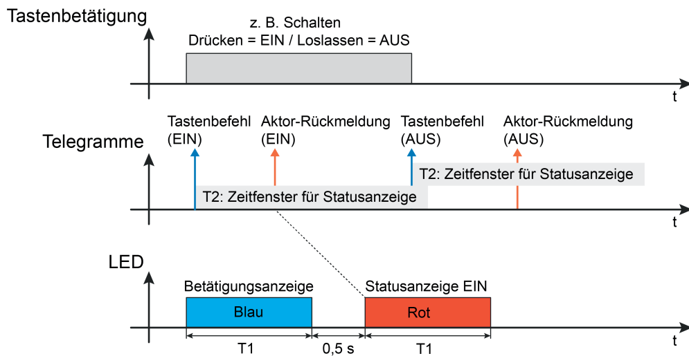
Bild 13: Beispiel einer Statusanzeige der Bedienfunktion "Schalten" Telegramm beim Drücken und Loslassen der Taste
