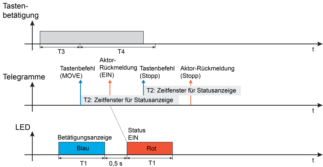
Bild 18: Beispiel einer Statusanzeige der Bedienfunktion "Jalousie" bei einem langen Tastendruck
