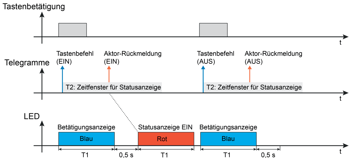
Bild 5: Beispiel einer 2-stufigen Betätigungs- und Statusanzeige Statusanzeige Zustand "EIN" durch rote LED
