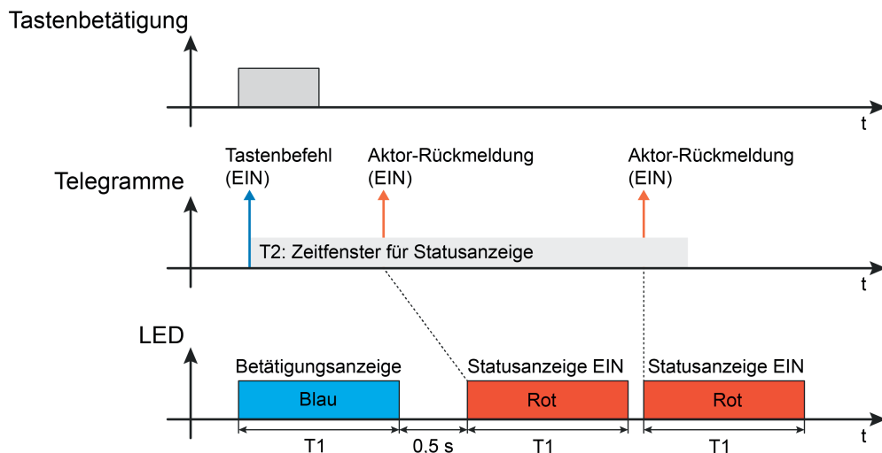
Bild 8: Beispiel einer 2-stufigen Betätigungs- und Statusanzeige bei zwei Aktor-Rückmeldungen Empfang zweier Aktor-Statustmeldungen im Zeitfenster zugelassen
