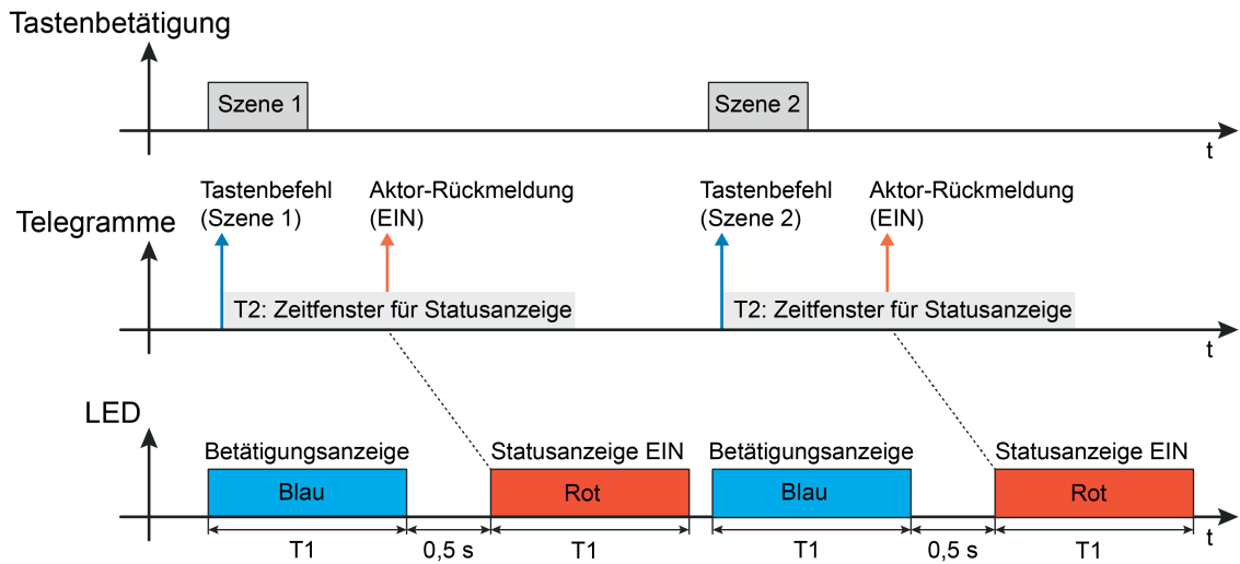
Bild 20: Beispiel einer Statusanzeige der Bedienfunktion "Szenennebenstelle" Szenennebenstelle ohne Speicherfunktion
