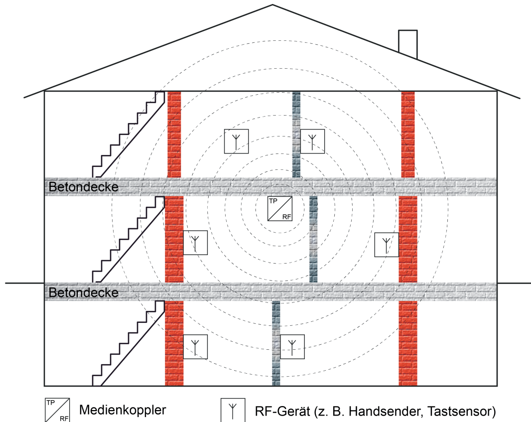
Bild 33: Gebäudestruktur mit einer KNX RF Linie (Beispiel)
