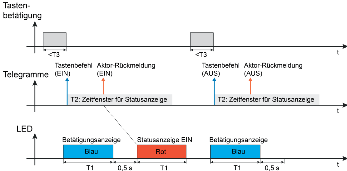
Bild 14: Beispiel einer Statusanzeige der Bedienfunktion "Dimmen" bei einem kurzen Tastendruck
