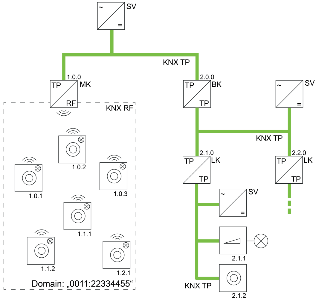
Bild 39: Beispiel einer möglichen KNX-Topologie mit RF- und TP-Linien Medienkoppler als Bereichskoppler
