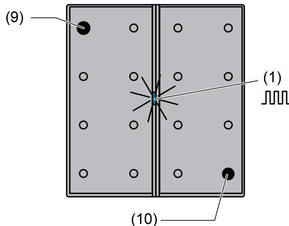
Bild 4: Tasten zur Aktivierung des Programmiermodus
