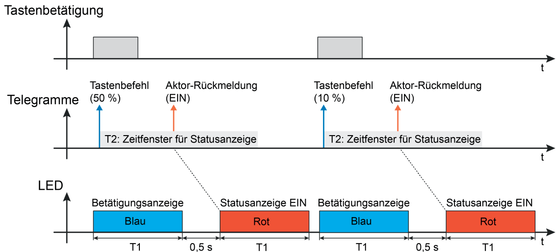
Bild 19: Beispiel einer Statusanzeige der Bedienfunktion "Wertgeber 1 Byte" Telegramm beim Drücken der Taste
