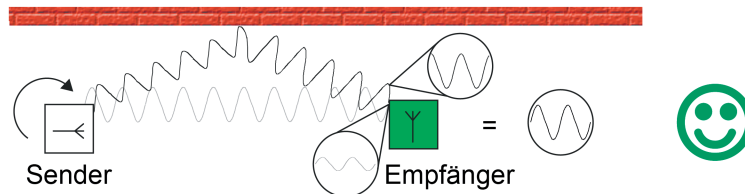
Bild 32: Reflexion ermöglicht Empfang durch Polarisationswechsel
