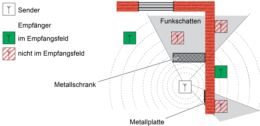
Bild 29: Funkschatten in einem Gebäude durch Metallteile (idealisiert)
