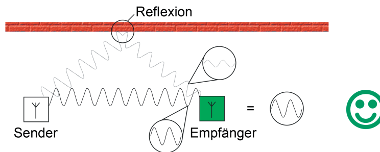
Bild 30: Interferenz beim Empfänger wirkungslos
