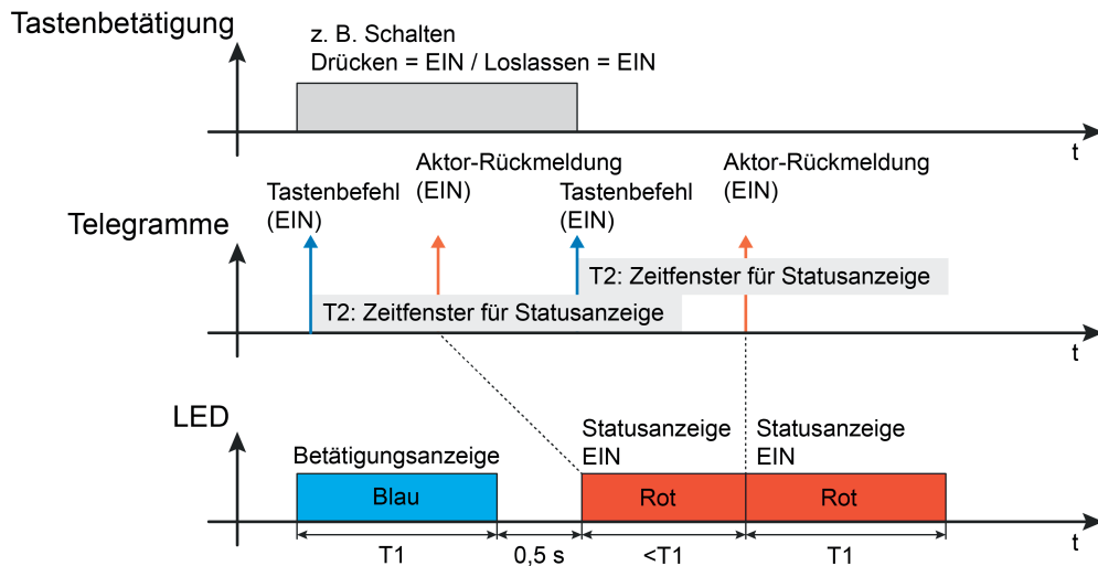
Bild 7: Beispiel einer 2-stufigen Betätigungs- und Statusanzeige bei zwei Aktor-Rückmeldungen Unterbrechung der ersten Statusanzeige durch Aktorstatus im neuen Zeitfenster
