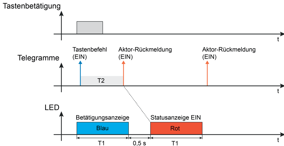
Bild 9: Beispiel einer 2-stufigen Betätigungs- und Statusanzeige bei zwei Aktor-Rückmeldungen Empfang zweier Aktor-Statusmeldungen im Zeitfenster nicht zugelassen
