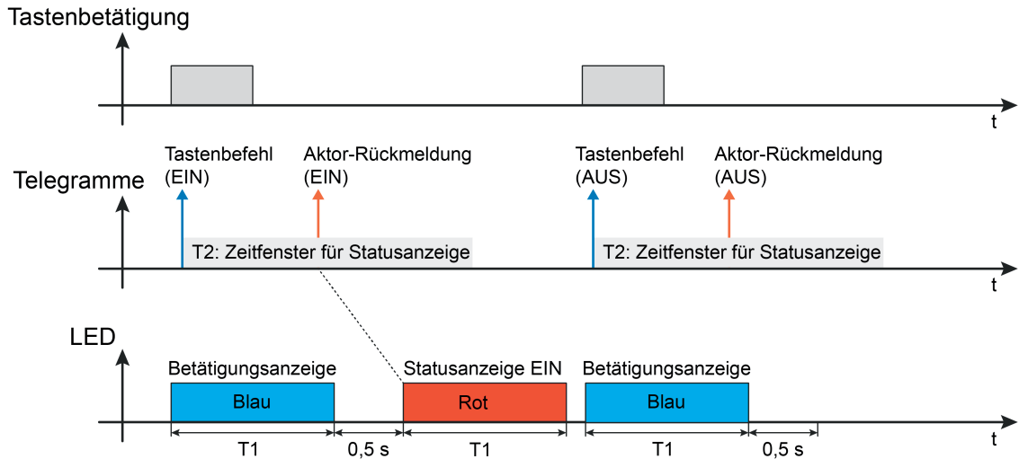
Bild 12: Beispiel einer Statusanzeige der Bedienfunktion "Schalten" Telegramm beim Drücken der Taste
