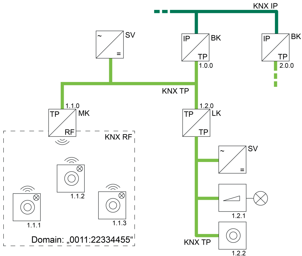
Bild 38: Beispiel einer möglichen KNX-Topologie mit RF-, TP- und IP-Linien Medienkoppler als Linienkoppler
