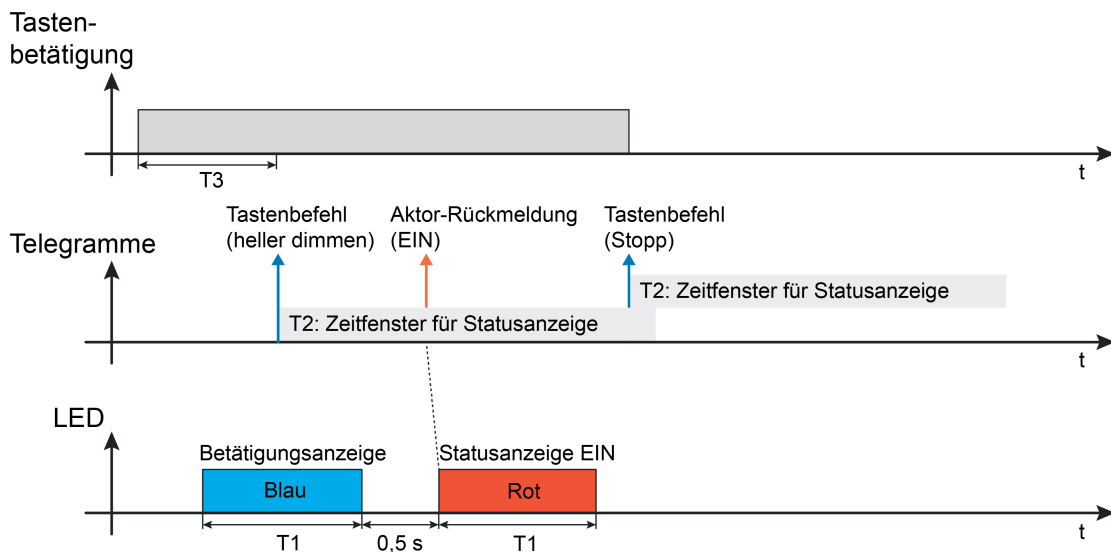
Bild 15: Beispiel einer Statusanzeige der Bedienfunktion "Dimmen" bei einem langen Tastendruck
