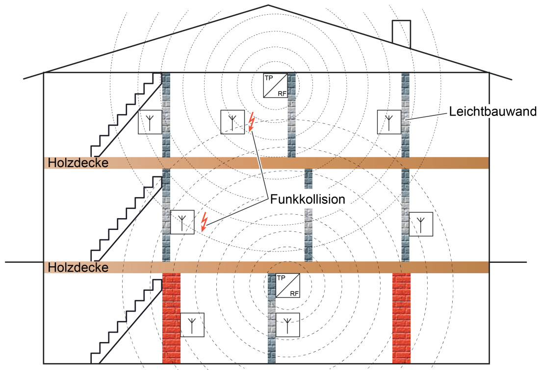
Bild 34: Gebäudestruktur mit zwei KNX RF Linien, ungünstige Beeinflussung (Beispiel)
