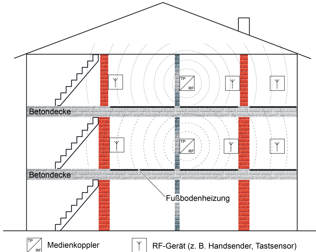
Bild 36: Gebäudestruktur mit zwei KNX RF Linien, die sich aufgrund der Gebäudebeschaffenheit nicht nachteilig beeinflussen (Beispiel)
