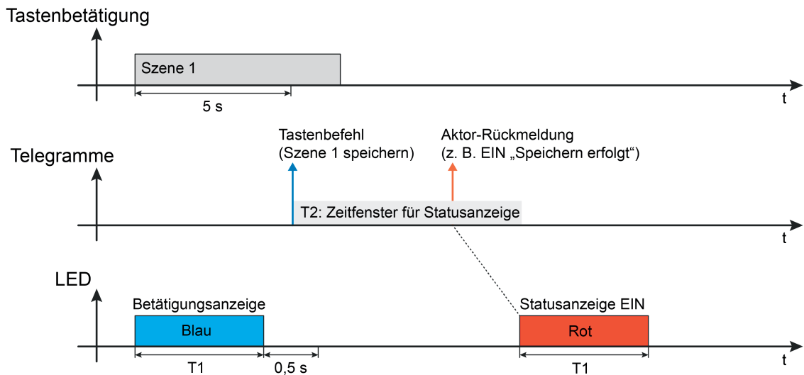
Bild 21: Beispiel einer Statusanzeige der Bedienfunktion "Szenennebenstelle" Szenennebenstelle mit Speicherfunktion und Statusanzeige
