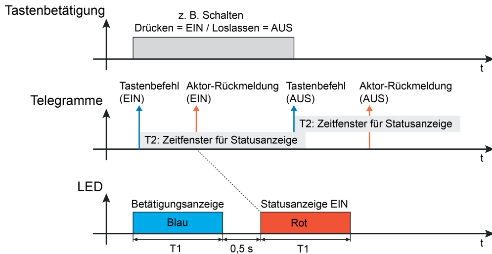
Bild 6: Beispiel einer 2-stufigen Betätigungs- und Statusanzeige bei zwei Aktor-Rückmeldungen Neue Zeitfenster für Statusanzeige durch mehrere Bedientelegramme
