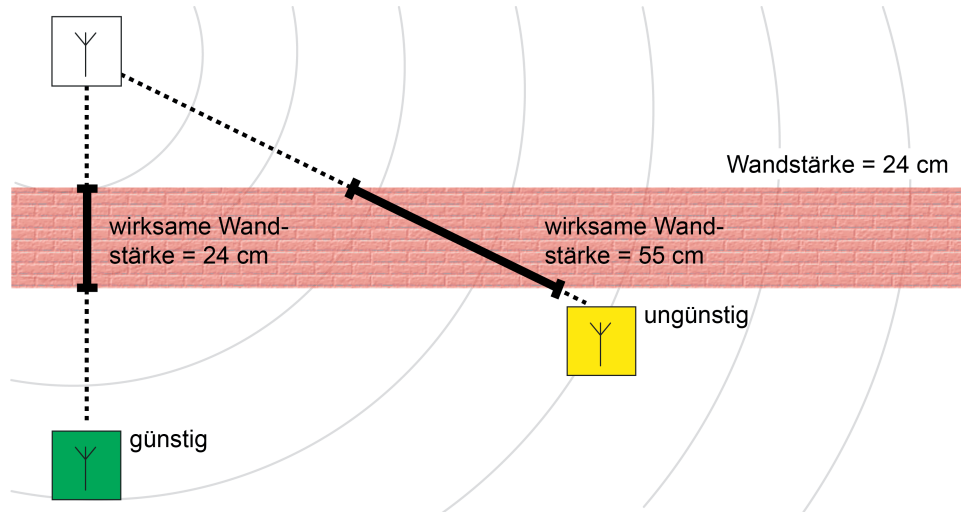
Bild 28: Dämpfung durch wirkungsvolle Wand- oder Deckenstärke
