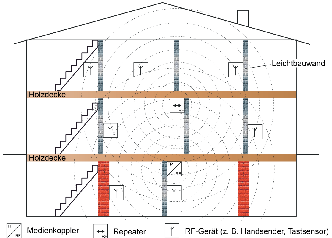
Bild 35: Gebäudestruktur mit einer KNX RF Linie und Repeater (Beispiel)
