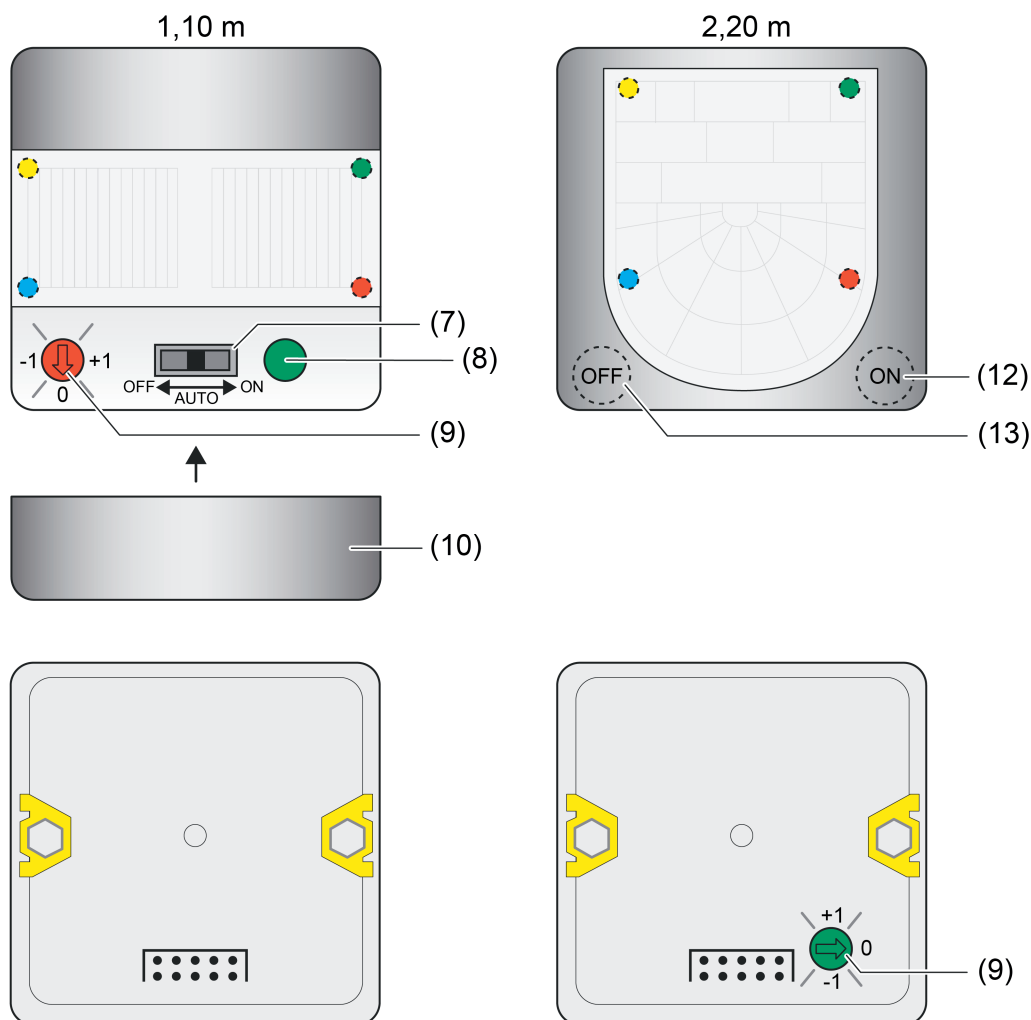
Bild 20: Bedienelemente am Gerät
