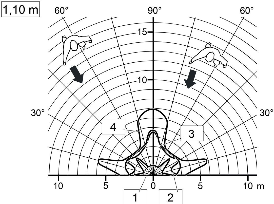
Bild 8: Reichweite bei radialer Bewegungsrichtung, Einbauhöhe 1,10 m
