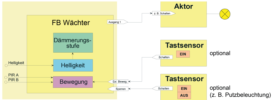
Bild 26: Applikationsbeispiel der Anwendung Wächter
