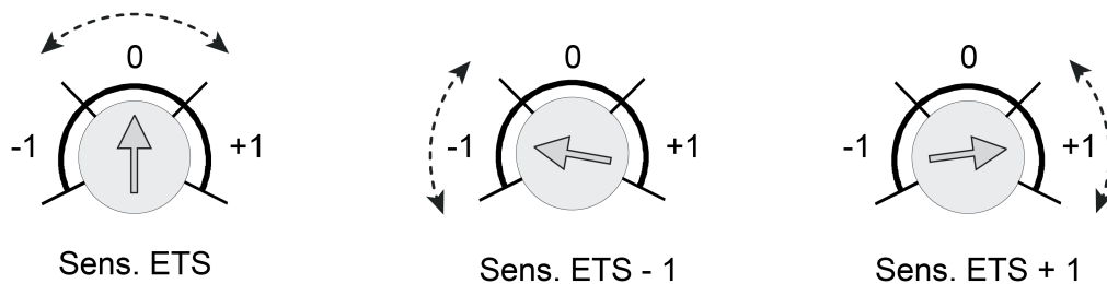
Bild 23: Beispiel zu den Einstellbereichen des Empfindlichkeitseinstellers am Gerät
