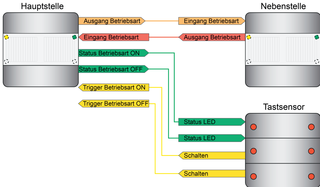
Bild 38: Beispiel zur Verknüpfung einer Hauptstelle mit einer Nebenstellen und einem Tastsensor zur Betriebsartenumschaltung und -anzeige
