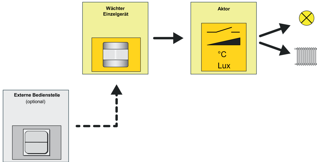
Bild 31: Applikationstyp "Einzelgerät"
