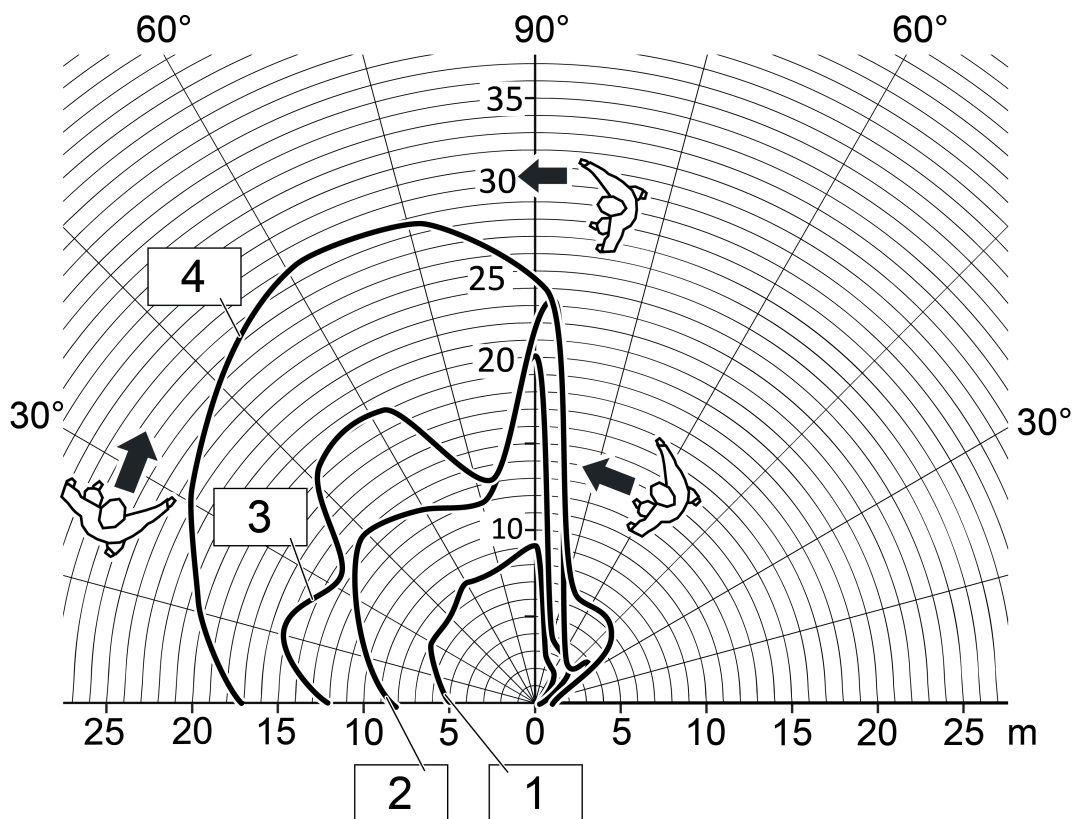
Bild 14: Reichweite bei tangentialer Bewegungsrichtung, Gerätevariante 1,10 m, nur ein Sensor aktiv
