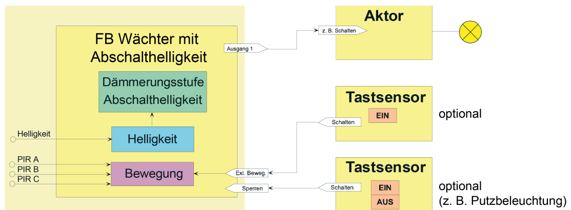
Bild 28: Applikationsbeispiel der Anwendung Wächter mit Abschalthelligkeit
