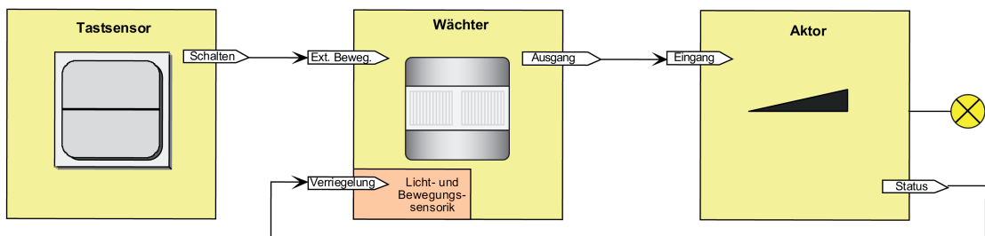
Bild 39: Applikationsbeispiel Einzelgerät mit externer Bewegungserfassung
