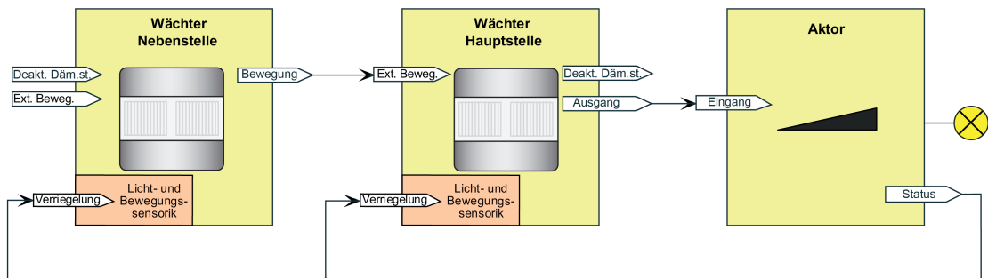
Bild 40: Applikationsbeispiel Haupt- und Nebenstelle ohne Dämmerungsstufenauswertung
