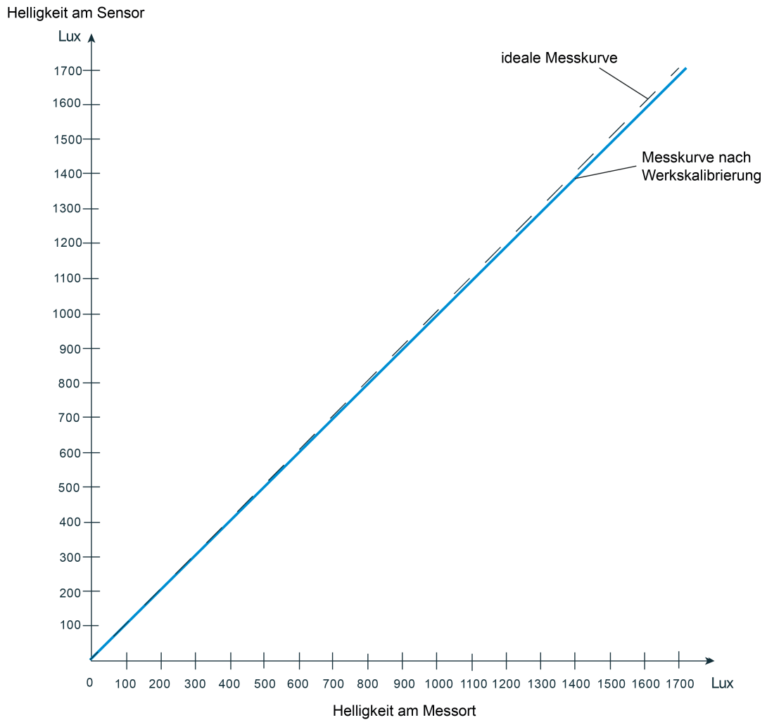
Bild 24: Messkennlinie nach Werkskalibrierung (Sensormesswert = Umgebungshelligkeit = ideale Messkennlinie)
