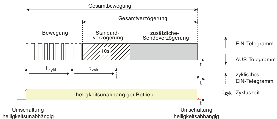
Bild 46: Gesamtbewegung mit Bewegungserfassung, Standardverzögerung und zusätzlicher Sendeverzögerung
