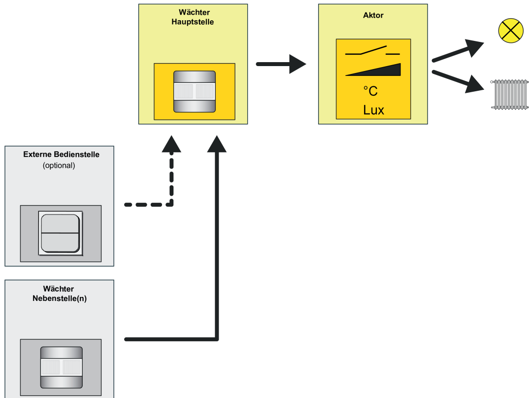
Bild 32: Applikationstyp "Hauptstelle"
