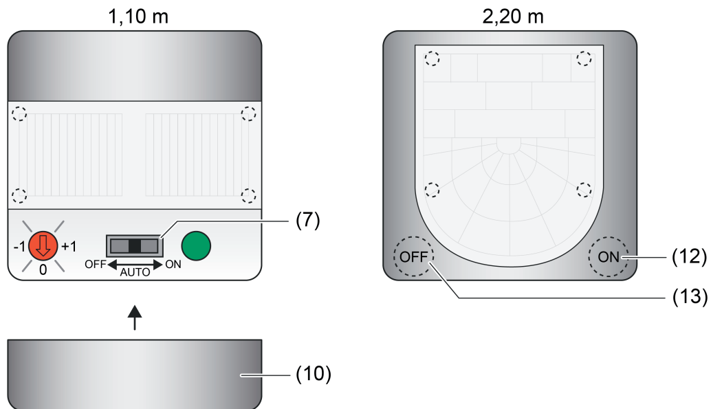
Bild 35: Anordnung der Bedienelemente zur Vor-Ort-Bedienung (Betriebsartenumschaltung)
