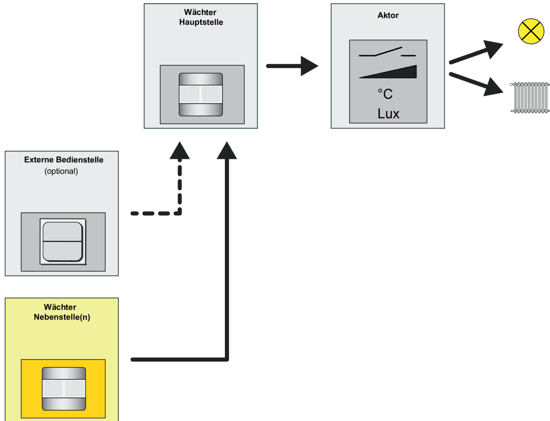
Bild 33: Applikationstyp "Nebenstelle"
