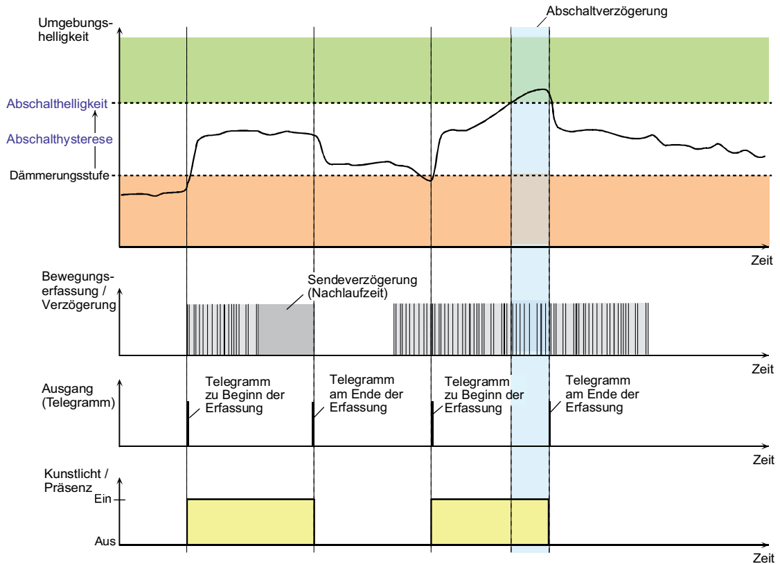
Bild 29: Helligkeits- und Bewegungsauswertung beim Wächter mit Abschalthelligkeit
