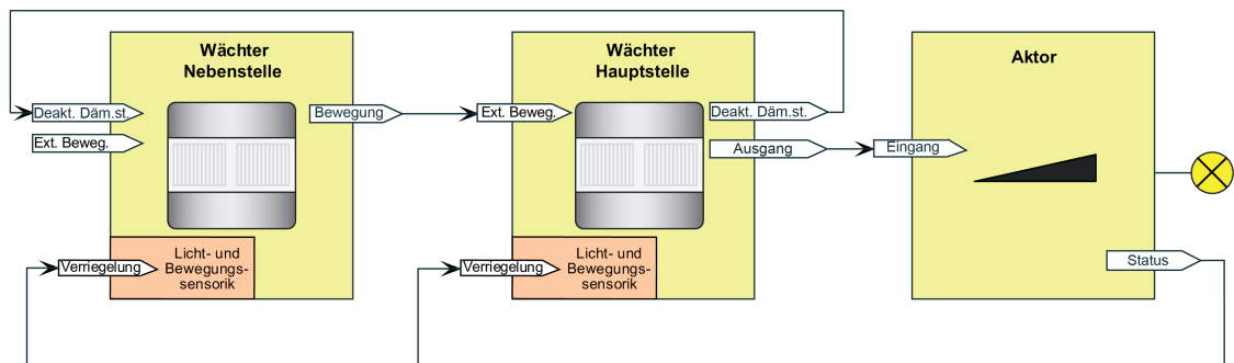
Bild 43: Applikationsbeispiel mit Dämmerungsstufenauswertung in der Hauptstelle und in den Nebenstellen Universal-Lösung für alle Datenformate
