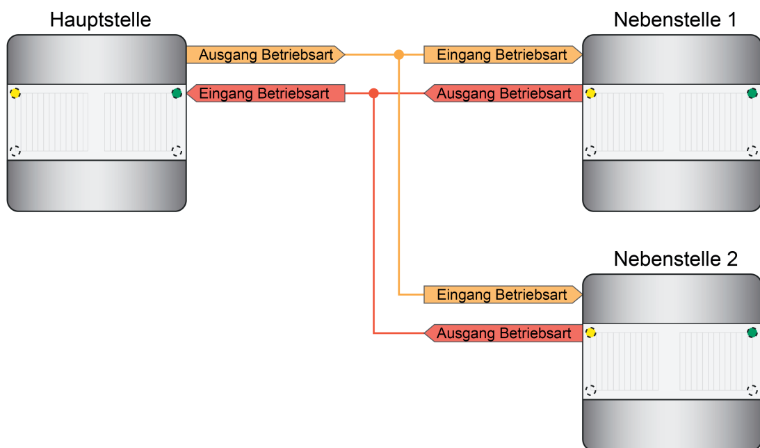
Bild 37: Beispiel zur Verknüpfung einer Hauptstelle mit zwei Nebenstellen zur Betriebsartenumschaltung und -anzeige
