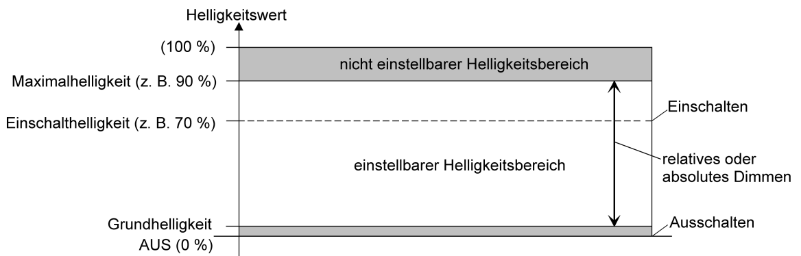
Bild 11: Beispiel eines Helligkeitsbereiches mit Grundhelligkeit
