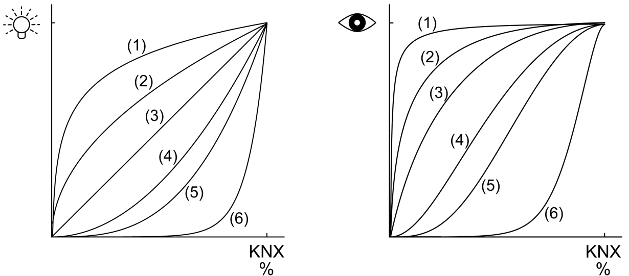
Bild 6: Dimmkennlinien im Wertebereich
