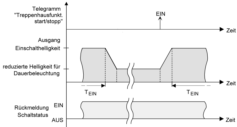
Bild 23: Die Dauerbeleuchtung der Treppenhausfunktion mit Soft-AUS-Funktion
