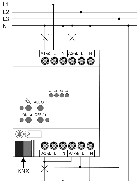
Bild 3: Geräteanschluss (Anschlussbeispiel)
