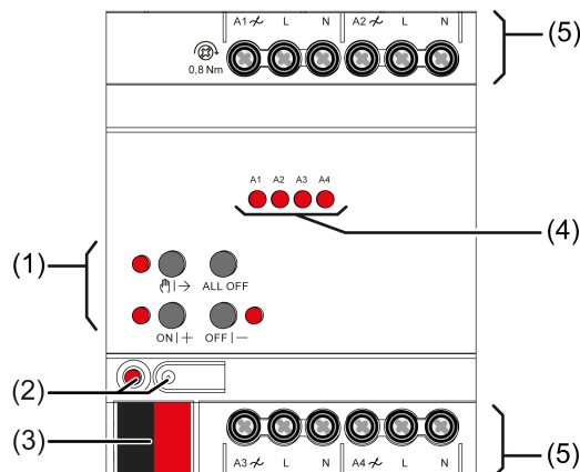
Bild 1: Geräteaufbau
