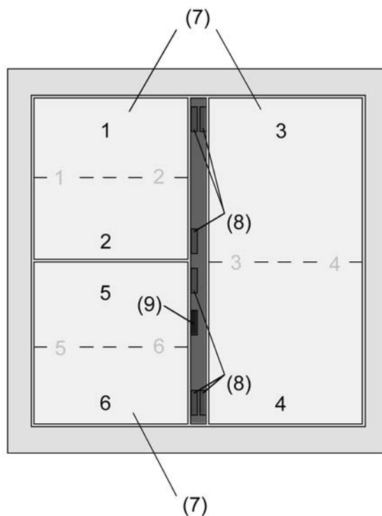
Bild 3: Geräteanordnung Tastsensor 3fach Universal TSM
