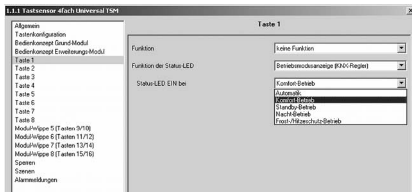
Bild 30: Parameteransicht für eine Status-LED als Betriebsmodusanzeige
