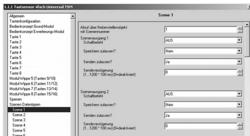
Bild 32: Parameteransicht für einzelne Szenenparameter
