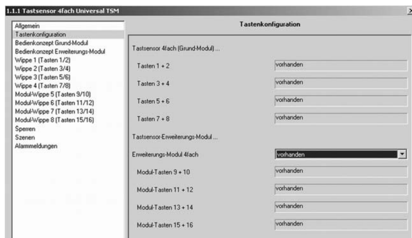
Bild 8: Parameteransicht für Tastenkongfiguration
