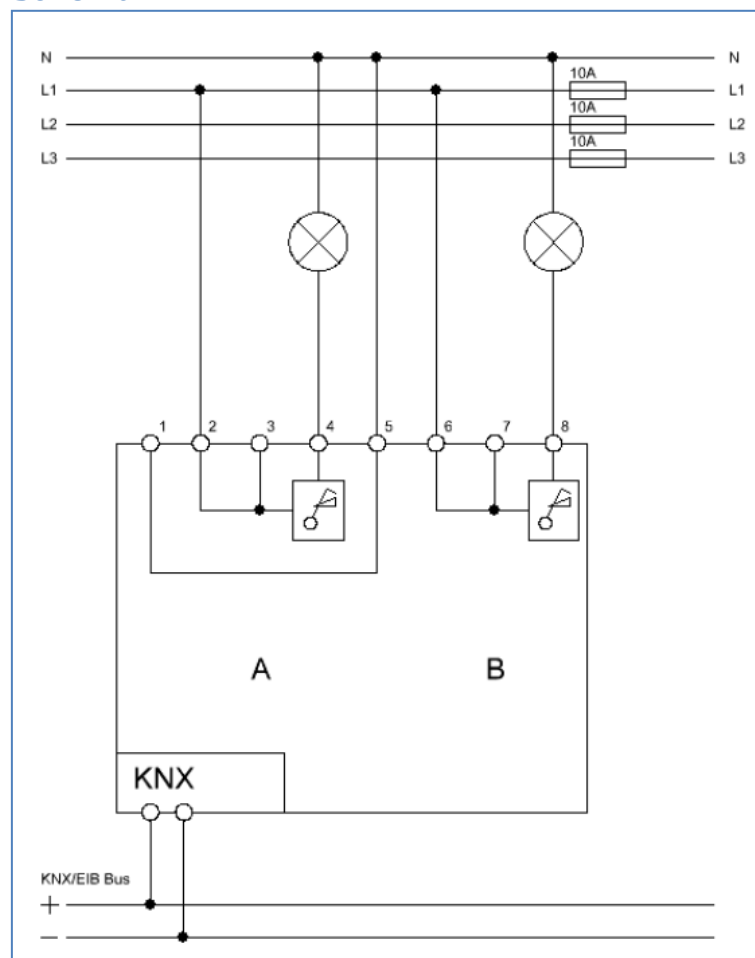
Bild 1: Anschluss-Schema AKD-0201.01
