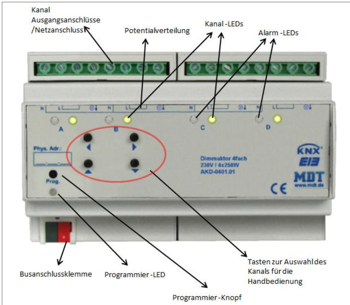
Bild3: Übersicht Hardwaremodul (AKD 0401.01)
