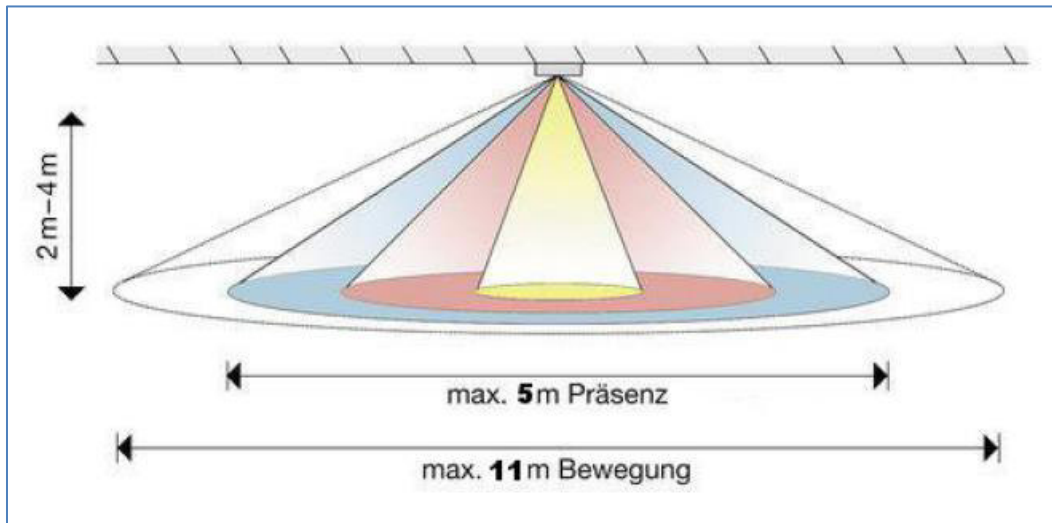
Abbildung 5: Erfassungsbereich SCN-P360x3.01
