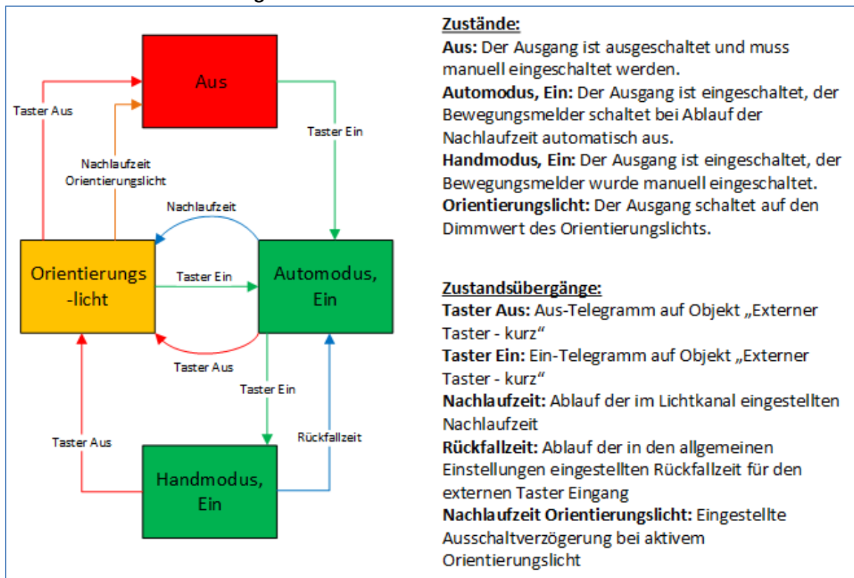
Abbildung 16: Halbautomat mit Orientierungslicht
