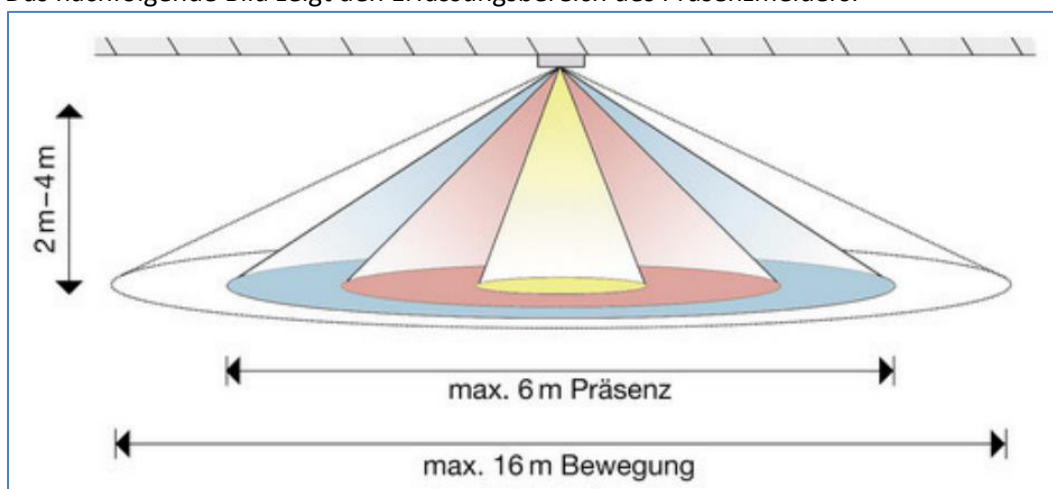
Abbildung 4: Erfassungsbereich SCN-P360x4.01
