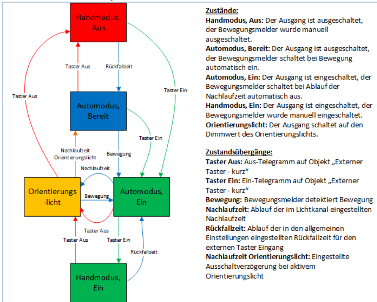
Abbildung 14: Vollautomat mit Orientierungslicht
