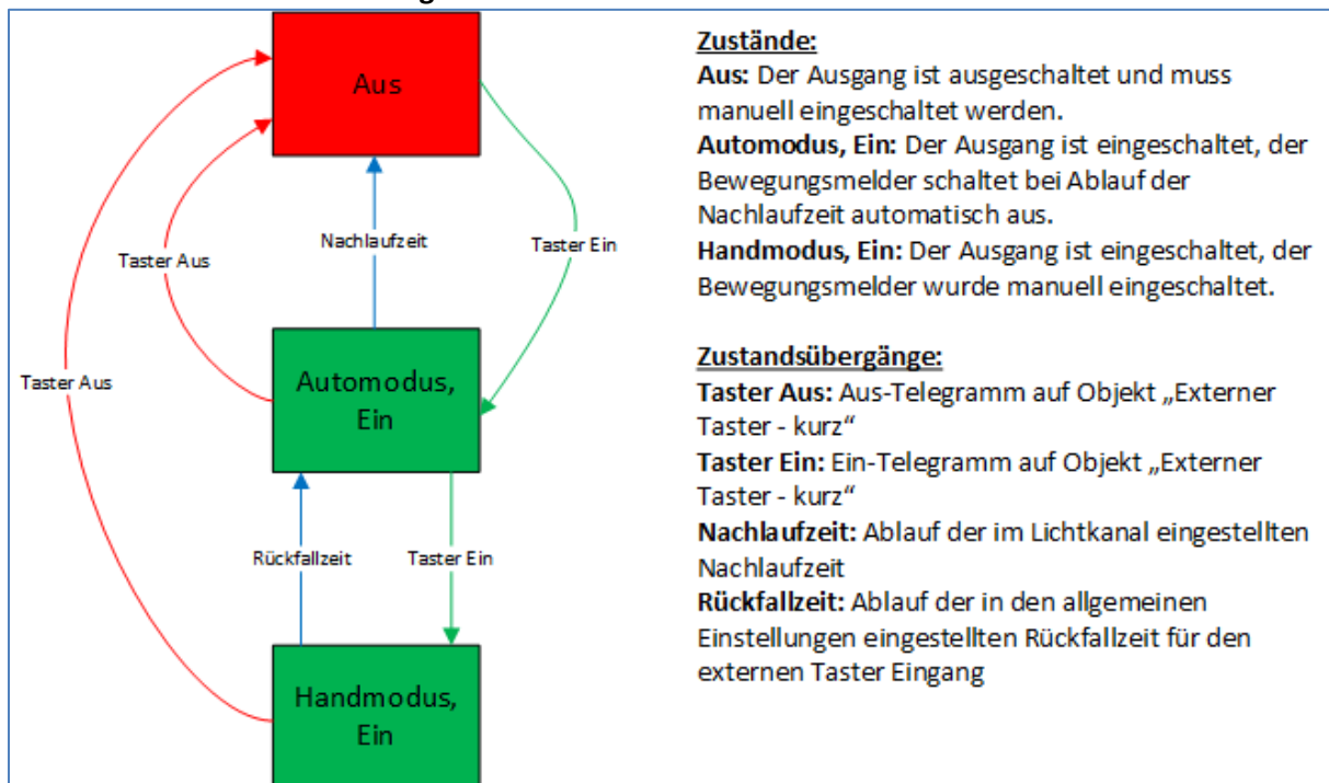
Abbildung 15: Halbautomat ohne Orientierungslicht
