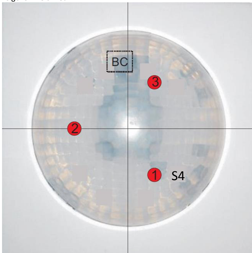
Abbildung 3: Anordnung der Sensoren und Leuchtdioden SCN-P/G360X3.01
