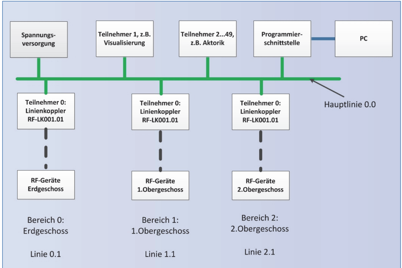
Abbildung 10: Topologie Beispielprojekt
