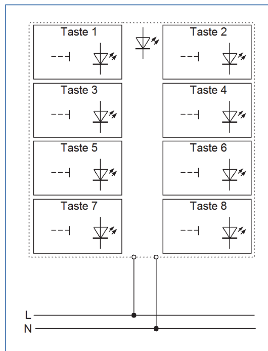
Abbildung 1: Anschlussbeispiel RF-TA55P8.01
