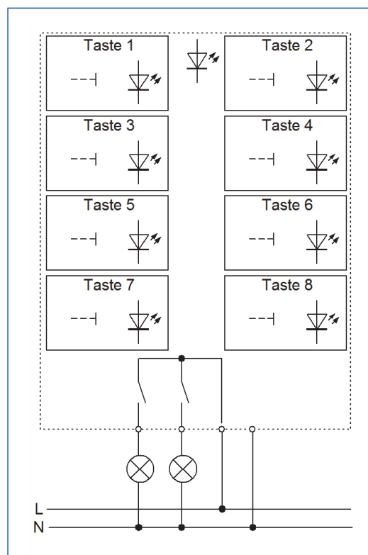
Abbildung 2: Anschlussbeispiel RF-TA55A8.01, mit Aktor
