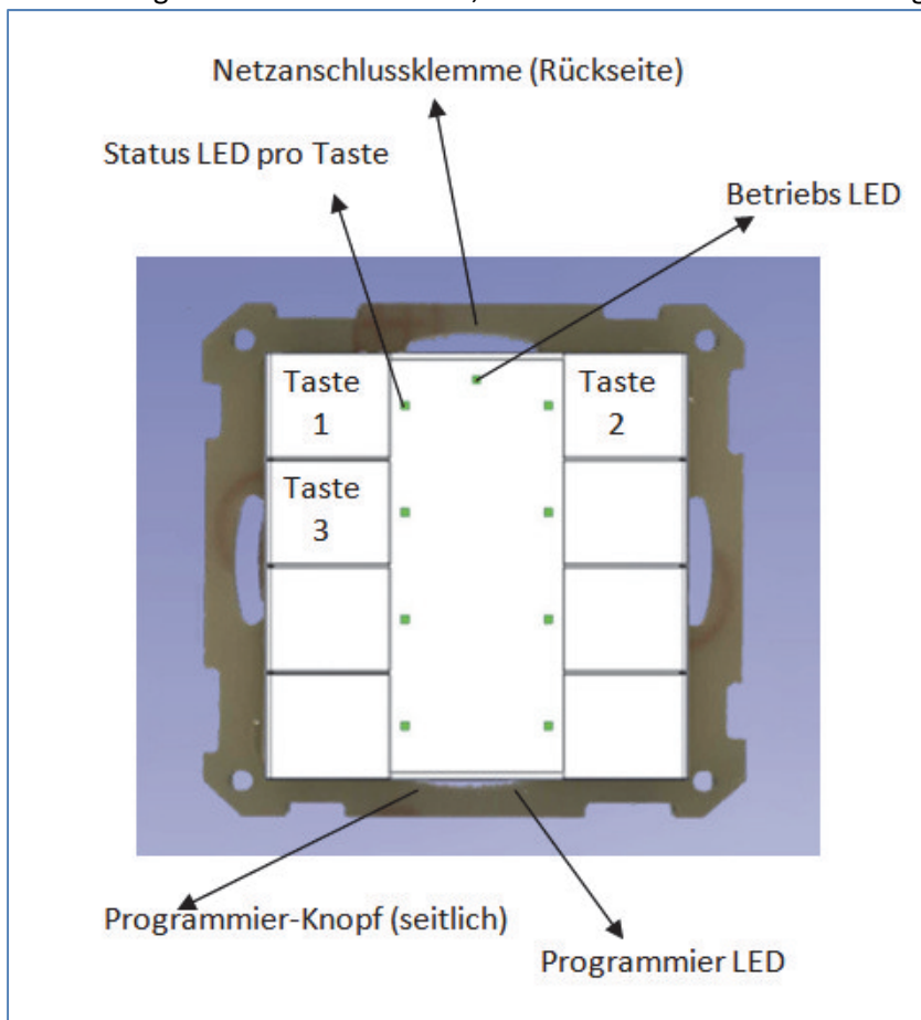
Abbildung 3: Übersicht Hardwaremodul Taster
