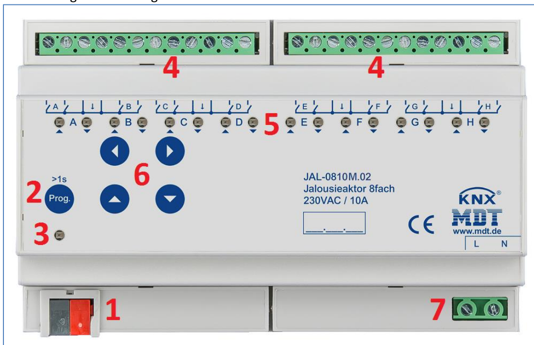
Abbildung 2: Übersicht Hardwaremodul (JAL-0810M.02)
