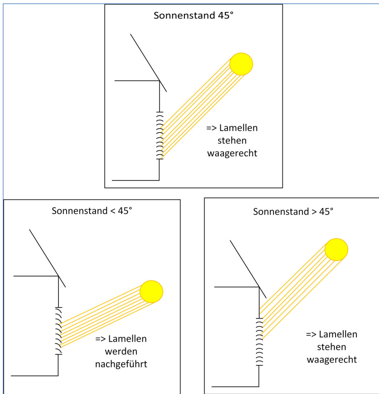
Abbildung 32: Grundprinzip Lamellennachführung
