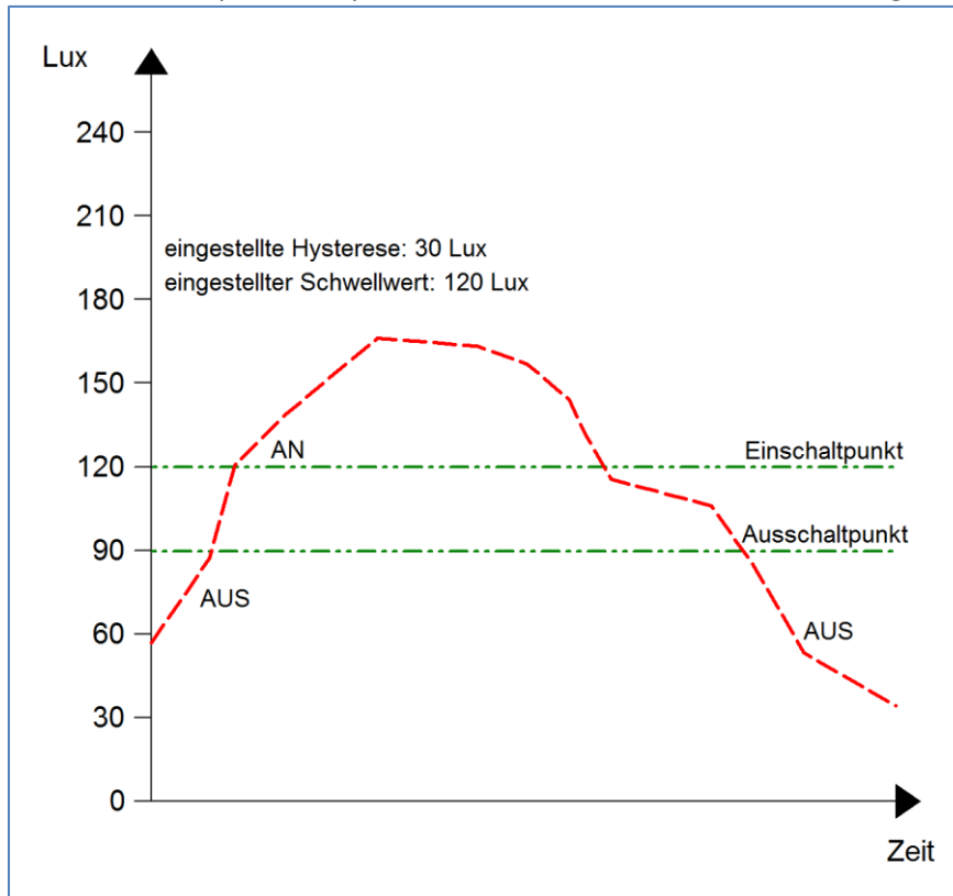
Abbildung 28: Beispiel – Schwellwertschalter/Hysterese
