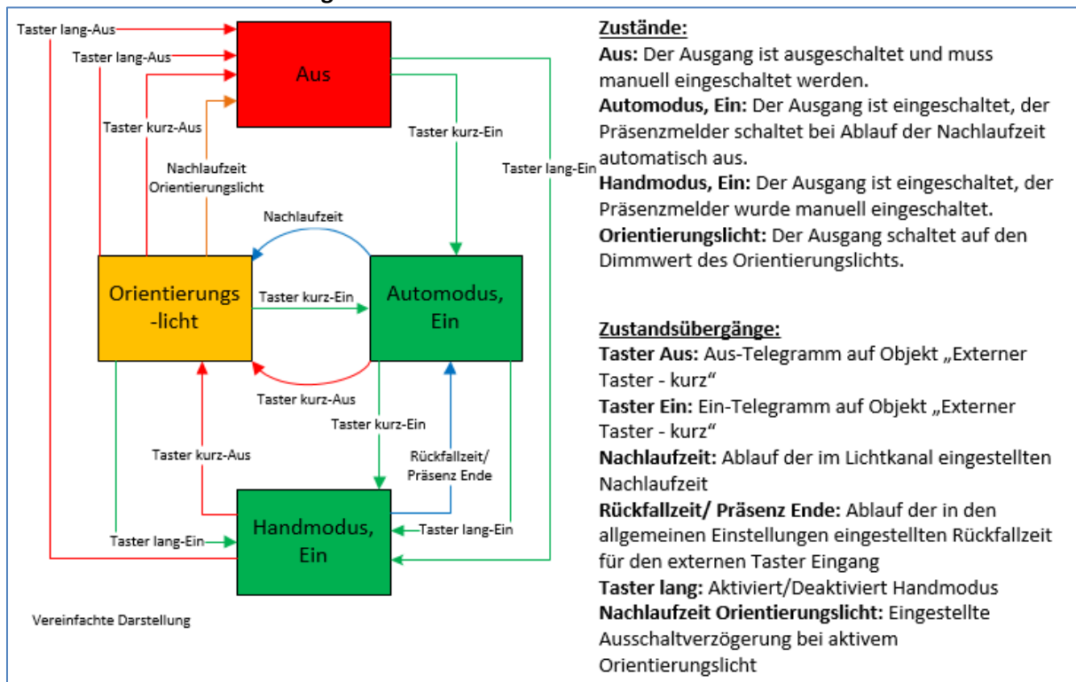
Abbildung 23: Ablaufdiagramm – Halbautomat mit Orientierungslicht
