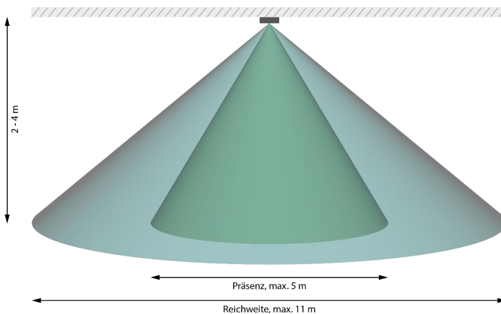
Abbildung 6: Erfassungsbereich SCN-x360x3.03
