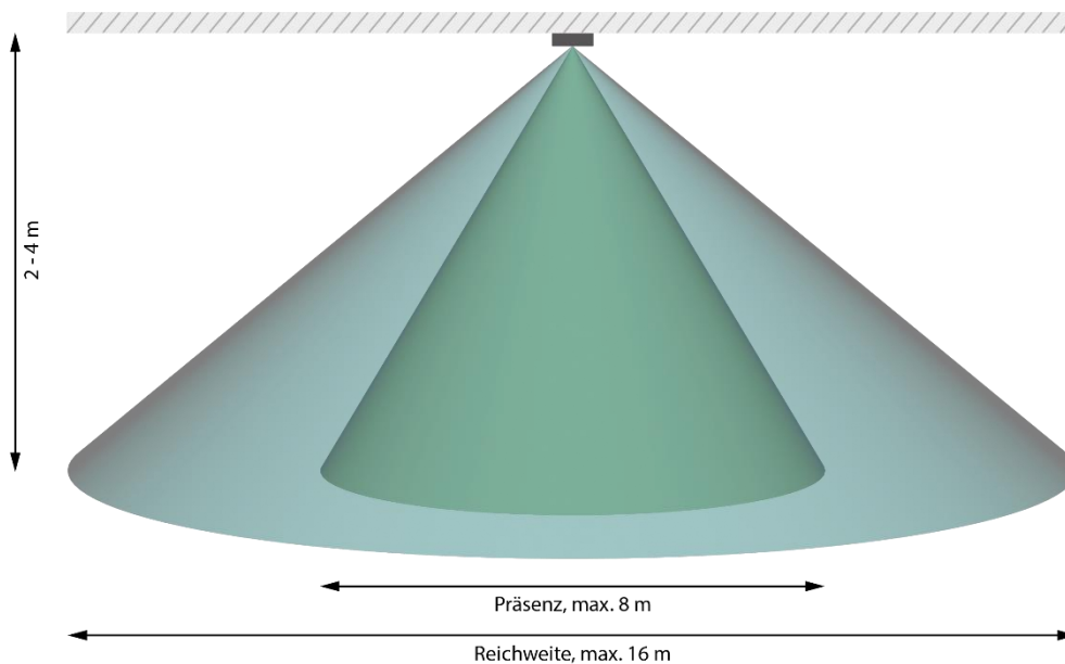
Abbildung 5: Erfassungsbereich SCN-P360x4.03
