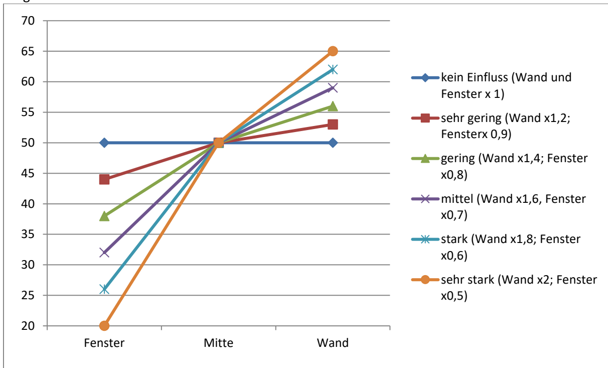
Abbildung 32: KLR – Einfluss Regelfaktoren
