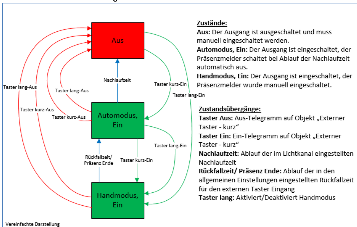
Abbildung 22: Ablaufdiagramm – Halbautomat ohne Orientierungslicht
