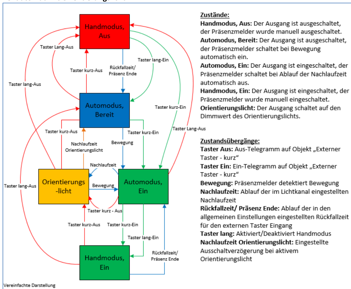
Abbildung 21: Ablaufdiagramm – Vollautomat mit Orientierungslicht
