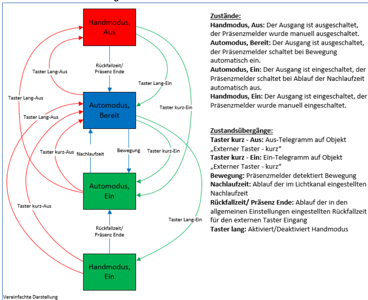
Abbildung 20: Ablaufdiagramm – Vollautomat ohne Orientierungslicht
