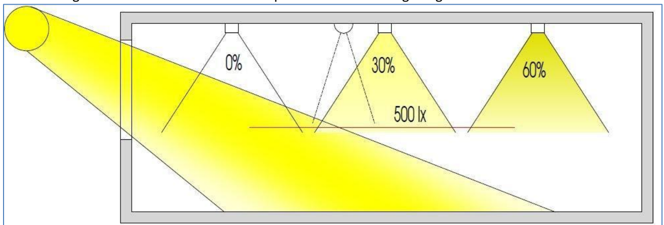
Abbildung 29: Funktionsprinzip – Proportionale Zonenregelung
