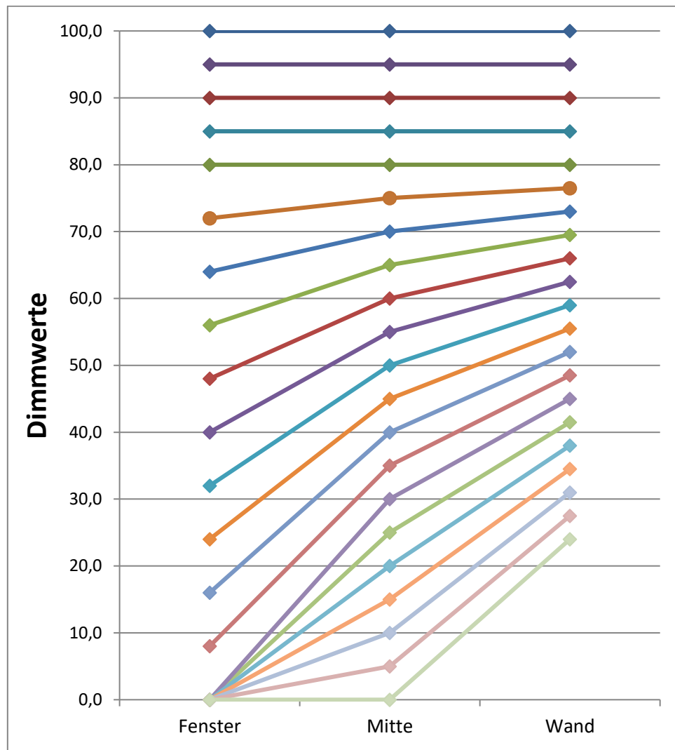
Abbildung 31: KLR – Verhalten proportionale Zonenregelung
