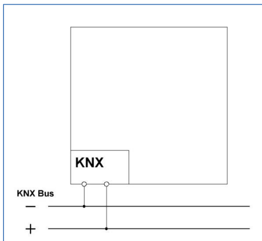
Abbildung 1: Anschluss-Schema
