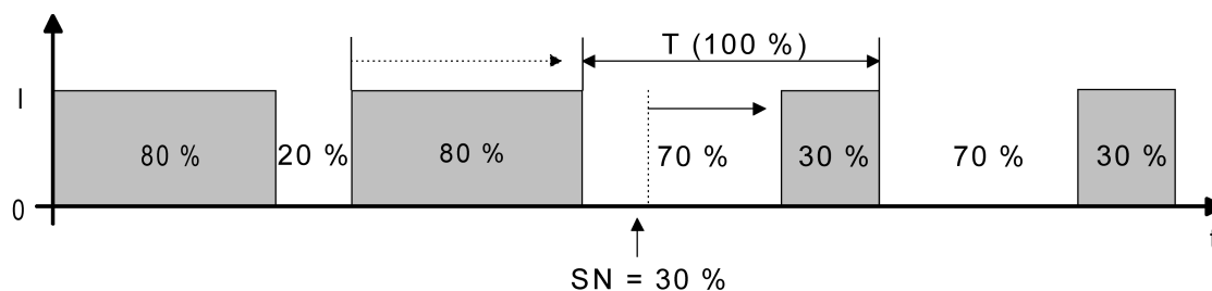
Bild 44: Stellgrößenänderung z. B. von 80 % auf 30 % während Schließphase des Ventils
