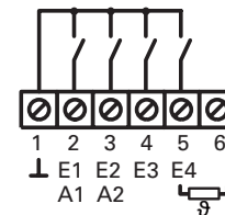
Bild 4: Schließen Sie die Binäreingänge an
