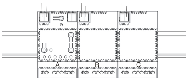
Bild 8. Verbinden von Universaldimmer-Erweiterungen
