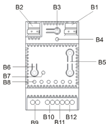
Bild 4. Anzeige- / Bedienelemente
