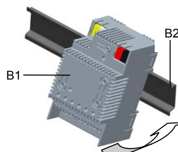
Bild 5. Montage auf einer Hutschiene
