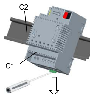
Bild 6. Demontage von einer Hutschiene
