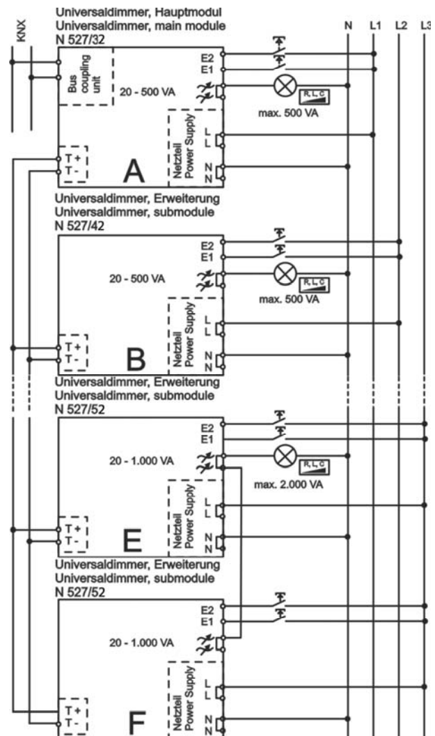
Bild 1. Anschlussbeispiel
