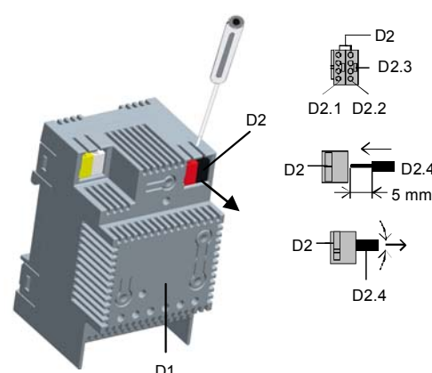
Bild 7. Klemmen aufstecken / entfernen
