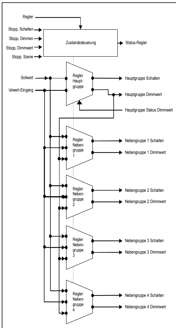
Abb. 27 Regleraufbau bei mehreren Leuchtgruppen
