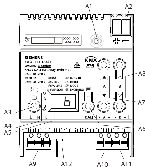
Abb. 39 Bedien- und Anzeigeelemente Gateway
