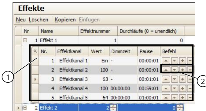
Abb. 21 Parameterfenster Effekte mit Effektschritte
