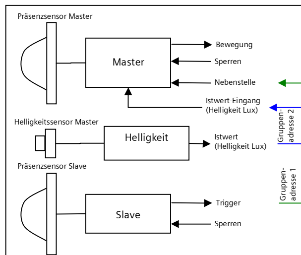
Abb. 15 Funktionsblöcke Hauptgerät=Master / Nebengruppe=Slave
