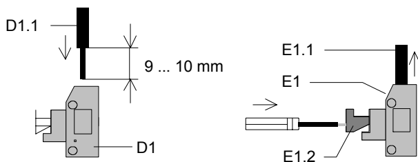
Bild 3: Leitungen anschließen und abklemmen
