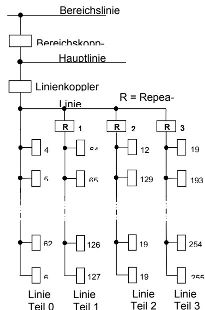
Bild 1. Anschluss von Repeatern an eine Linie
