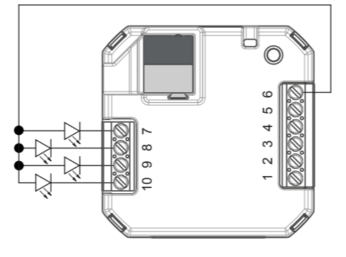
Collegamento uscite (LED a basso consumo)
