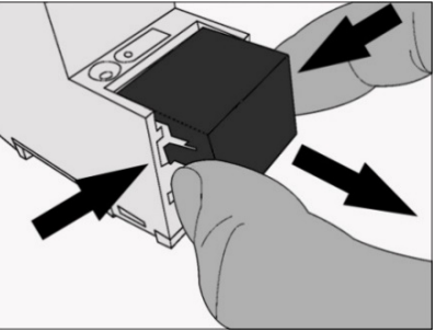
Abbildung 3: Abdeckkappe entfernen Figure 3: Remove the cover cap Afbeelding 3: Afdekkap verwijderen Figura 3: Rimozione del cappuccio di protezione Figura 3: Retirada de la caperuza de cubierta Illustration 3: Enlever le capuchon
