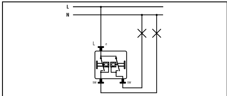
Wiring diagrams 535 U5
