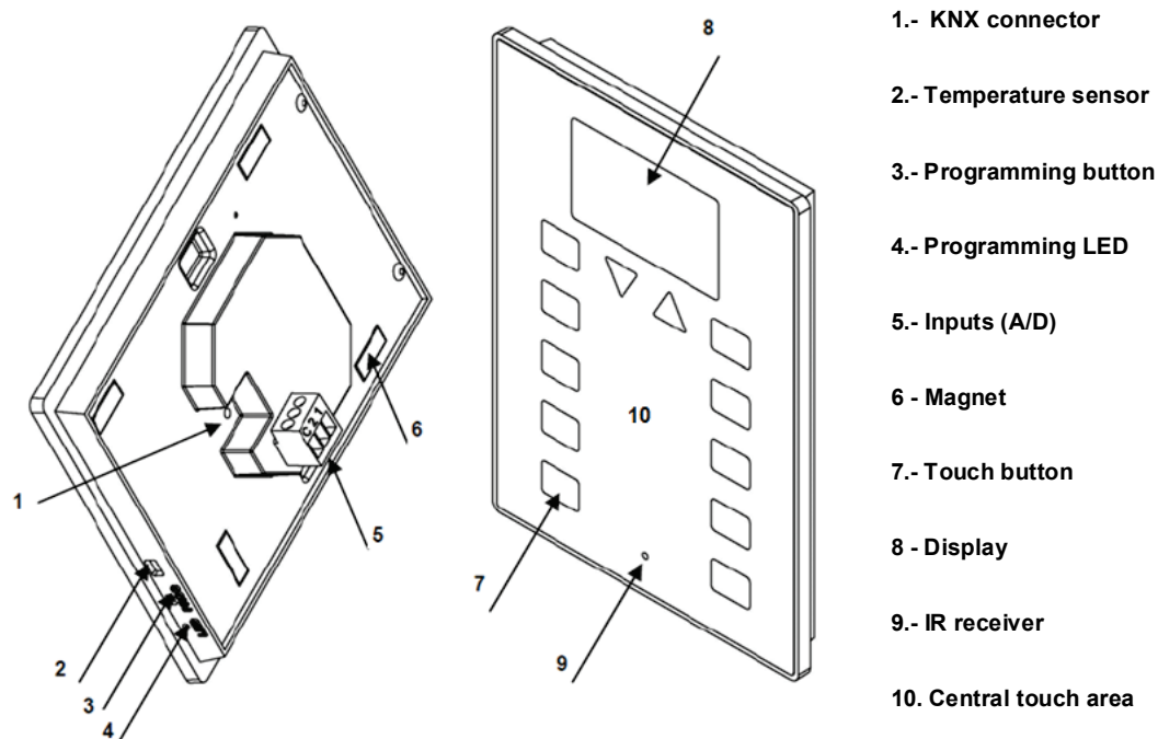
Figure 2. ZAS. Element diagram.
