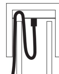
Fig. 10b: Sección del zócalo. Conducir el conductor entre el zócalo y el mástil hacia fuera
