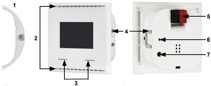
Fig. 1 1 Soporte de montaje con tornillos 2 Orificios para la circulación del aire 3 Teclas táctiles 4 Pestañas 5 Borne KNX BUS +/- 6 LED de programación (hundido) 7 Tecla de programación (hundida)
