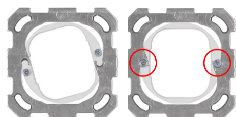
Fig. 2 Enganche el soporte de montaje en la placa de montaje del sistema de interruptores y apriete los tornillos.
