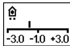
Fig. 8 Pantalla de modo con indicación analógica, área y número. Indicación de la zona de modificación posible (predefinida como en ETS) y de la modificación del valor teórico configurado. En el ajuste del regulador de la figura se ve "Valor teórico básico reducido 1,0°".
