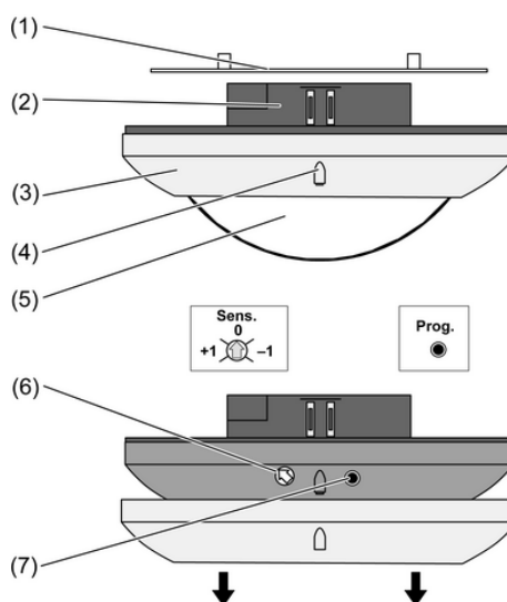
Figura 1: Estructura del mecanismo
