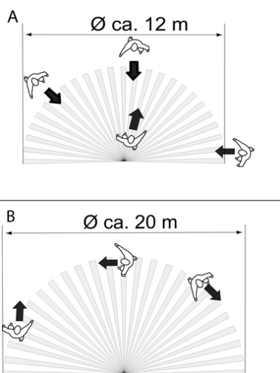
Figura 3: El alcance de la detección depende de la dirección del movimiento con una altura de montaje de 3 m
