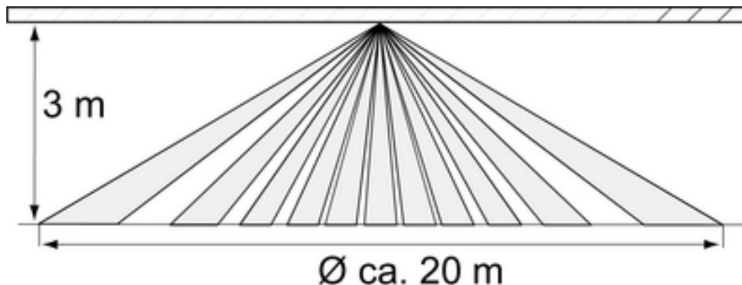
Figura 2: Ventana del sensor y área de detección
