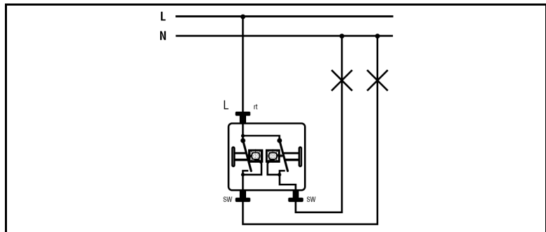
Ejemplos de conexionado 535 U5
