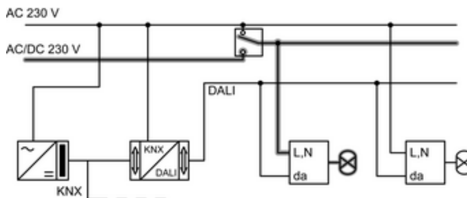
Figura 4: Lámparas de emergencia alimentadas mediante suministro central de seguridad
