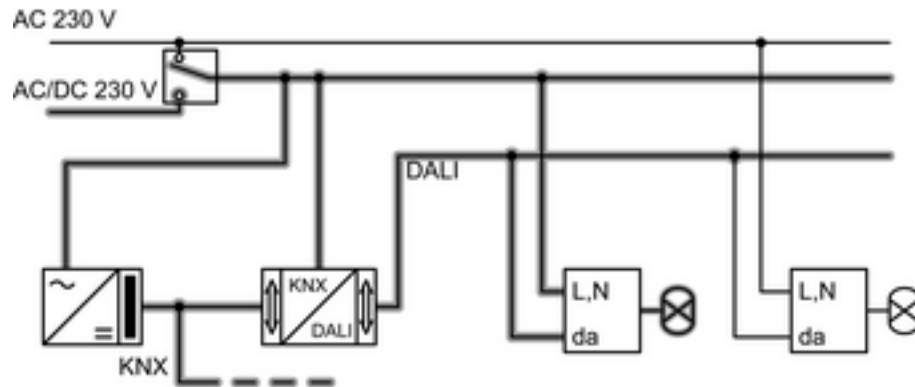
Figura 5: Lámparas de emergencia, instalación KNX y pasarela DALI alimentadas mediante suministro central de seguridad
