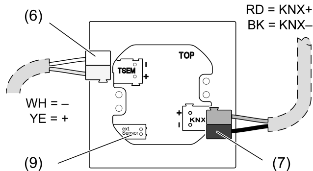
Imagen 4: Vista trasera del módulo Controlador de estancia
