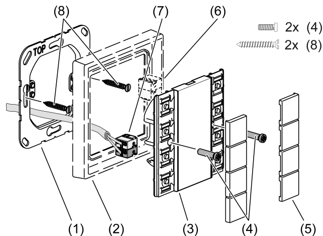
Imagen 3: Montaje del módulo Controlador de estancia
